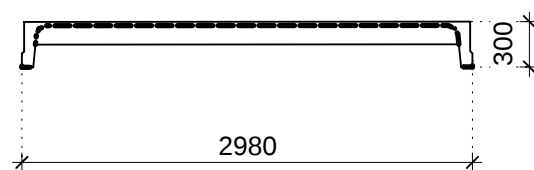
ПГЗХ6 Плита ребриста 64 штук
