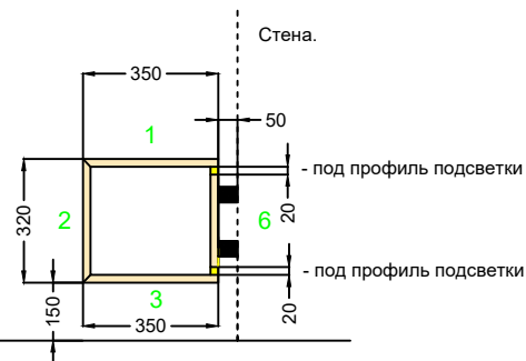
Размеры. Вид сбоку.
