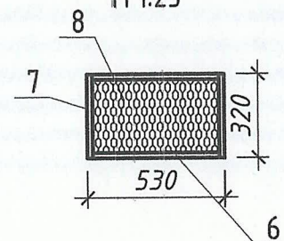
Конструкція сходинки М 1:25
