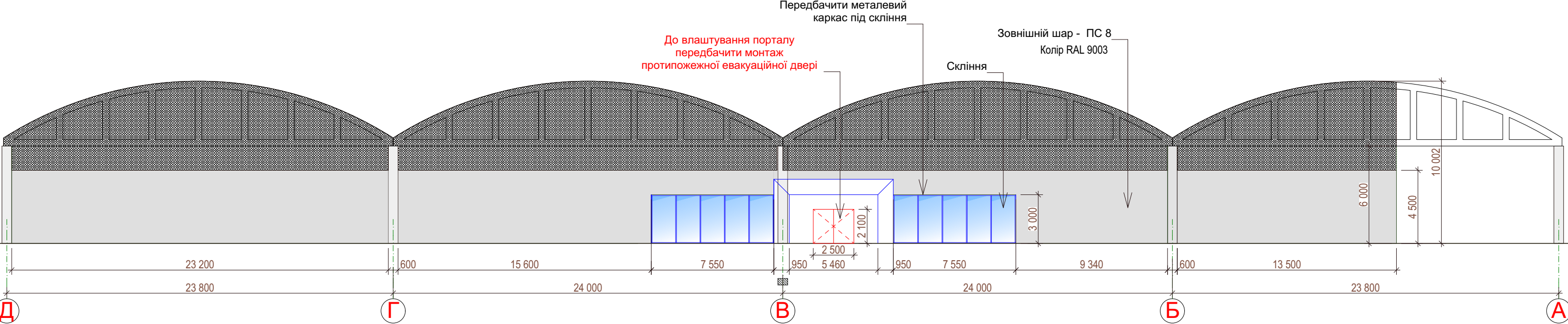
Вид А перегородки по осі 17 у вісях Д - А
