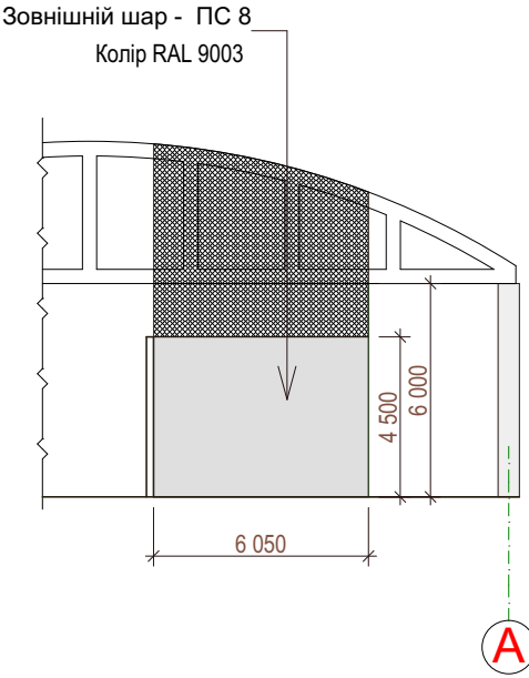
Вид С
