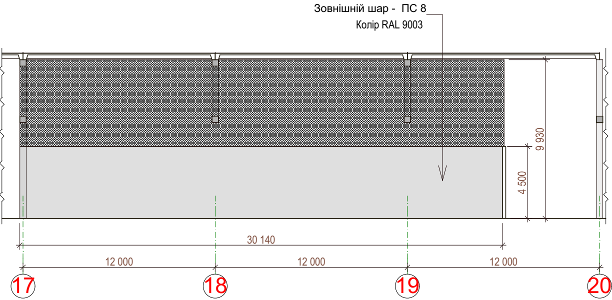
Вид В перегородки між осями Б-А1 у вісях 17 - 20
