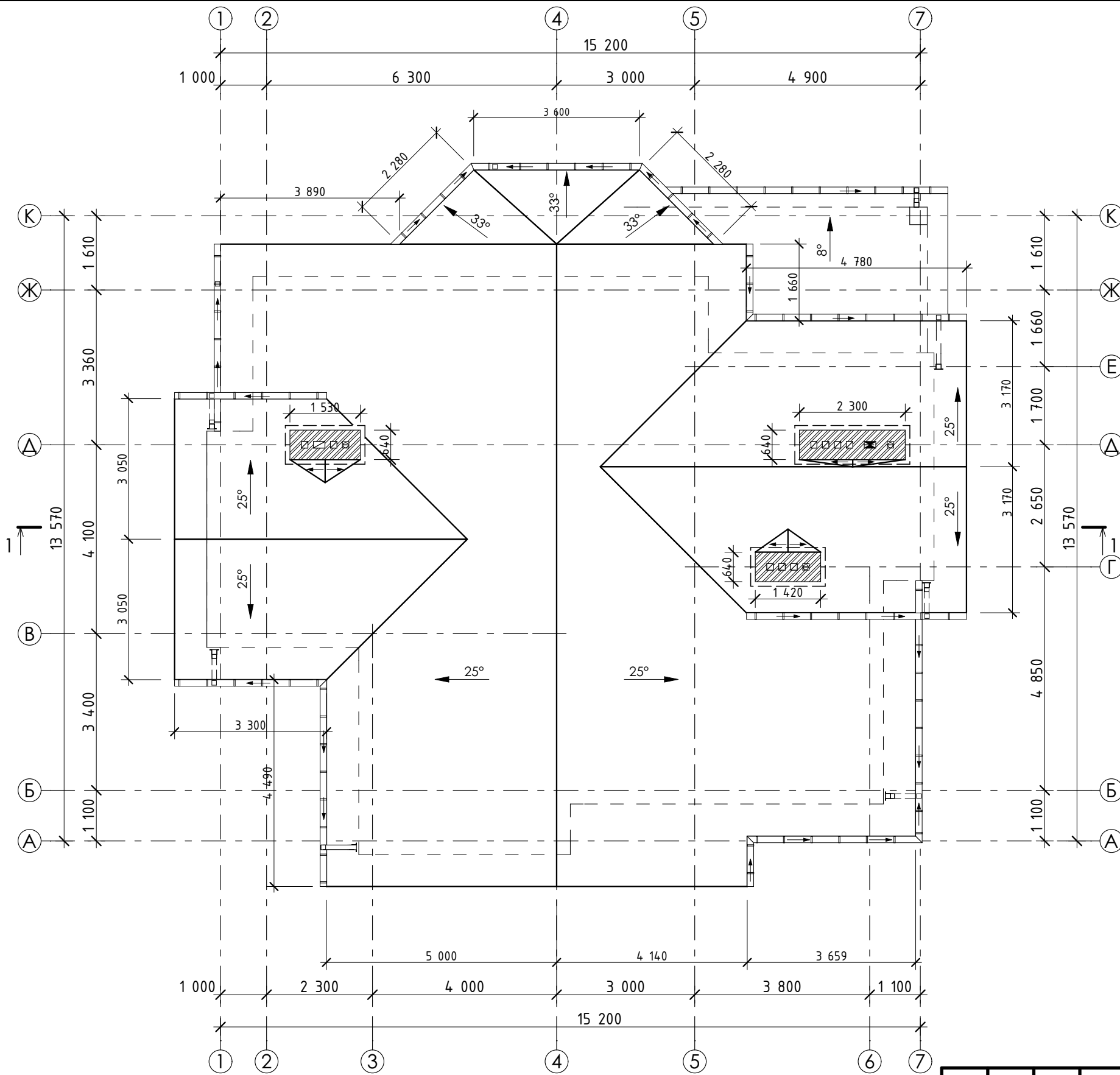
План покрівлі
