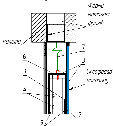
Вузол 1
