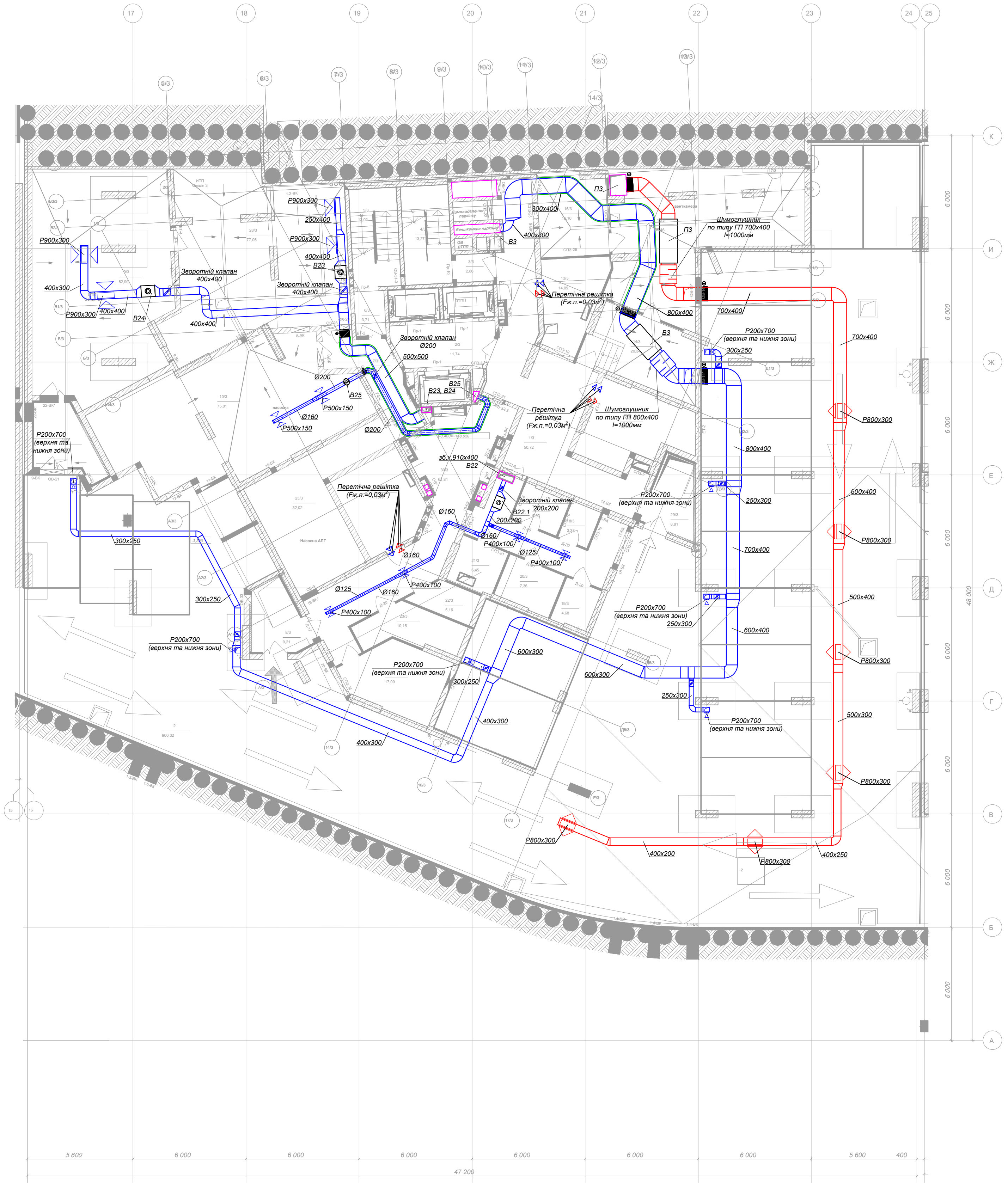
План -1 поверху на відм.-3,400
