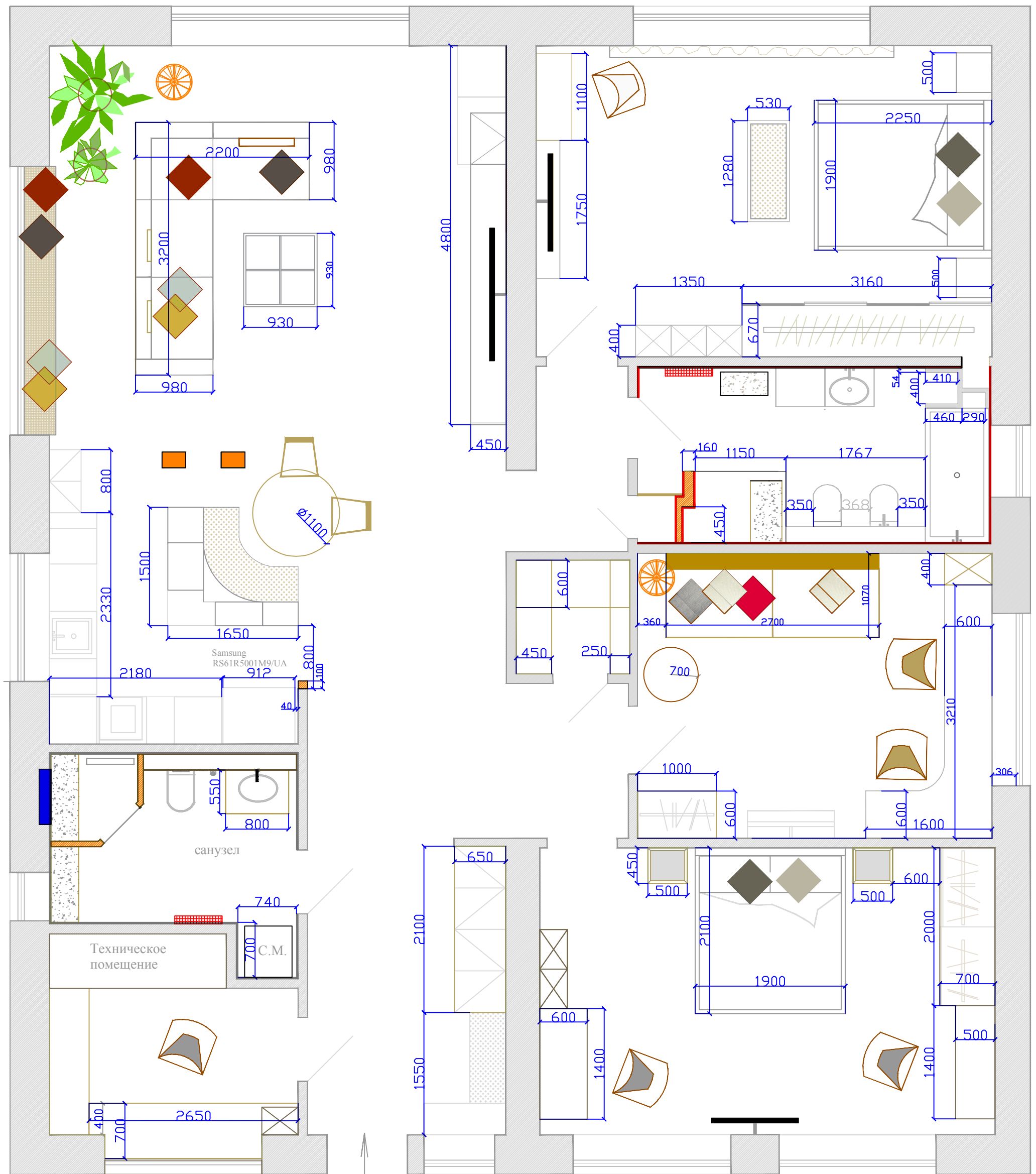
План с мебелью
