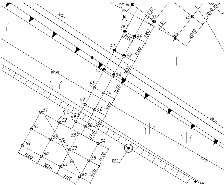
Схема розташування паль під пірс
