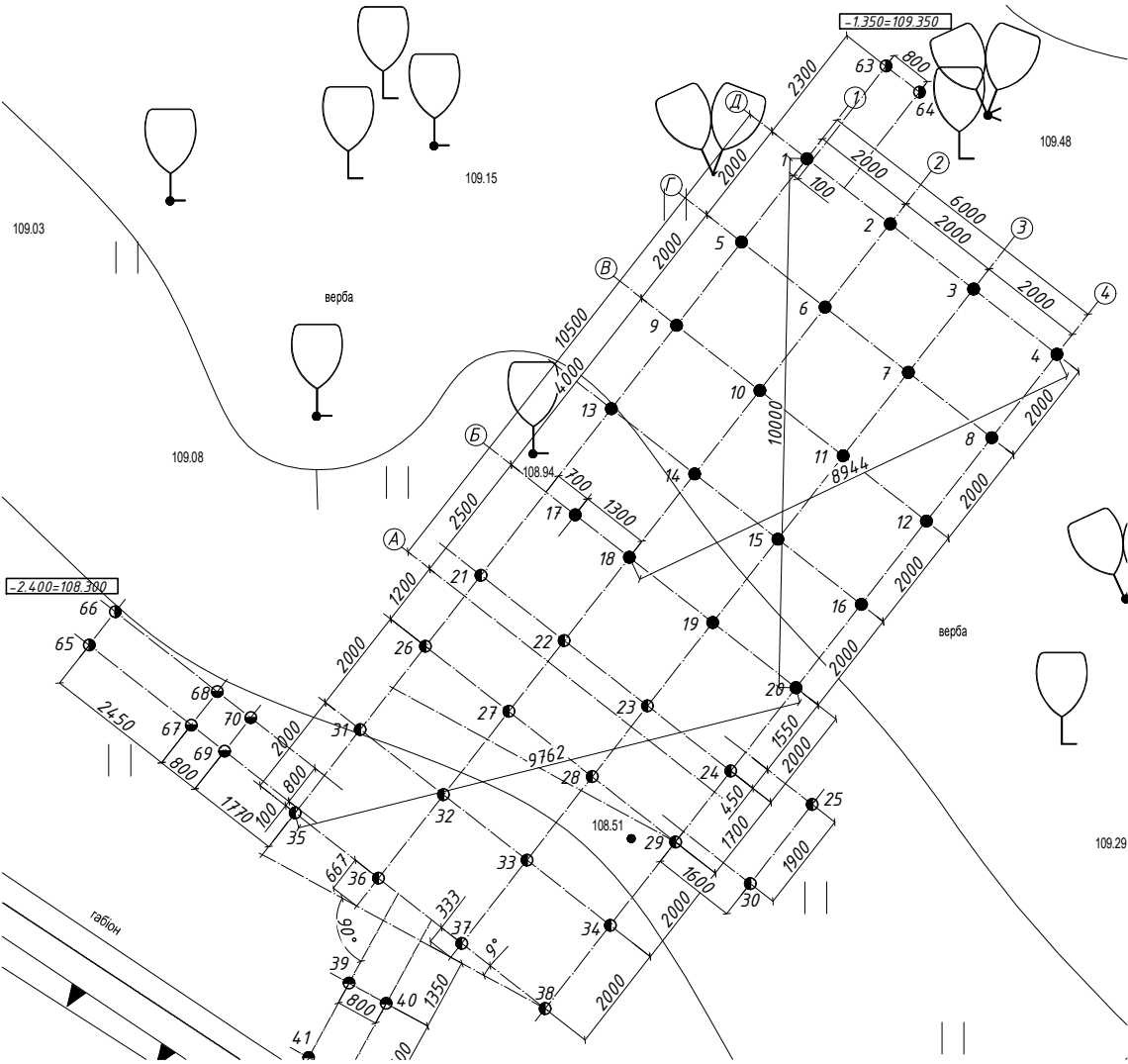
Схема розташування паль під будинок та оглядовий майданчик
