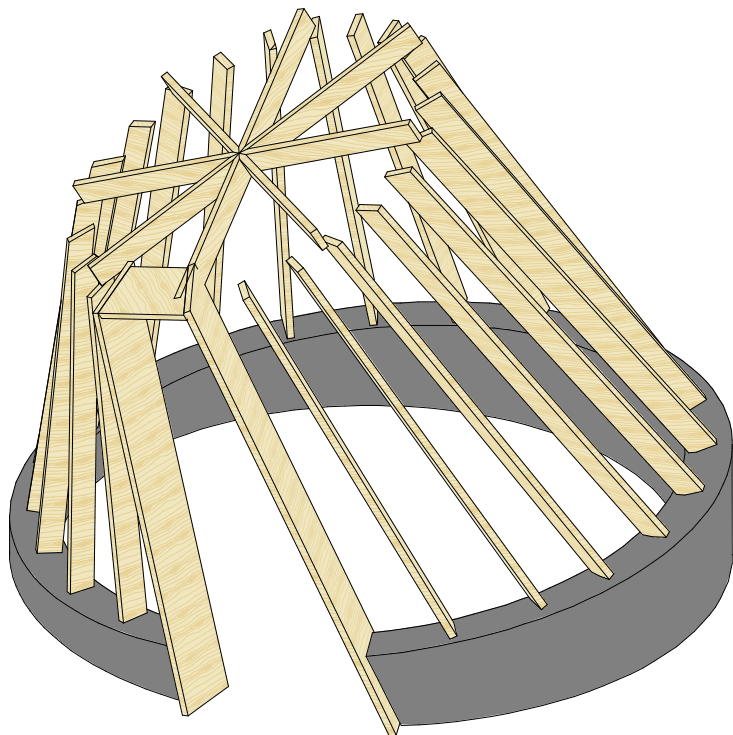
Каркас без оболонки
