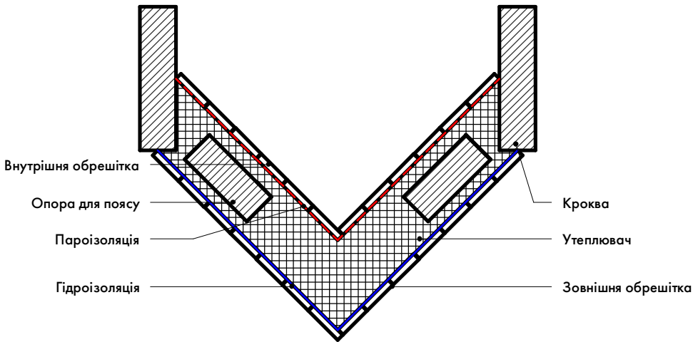
Вузол конструктивної схеми оболонки 1 : 15
