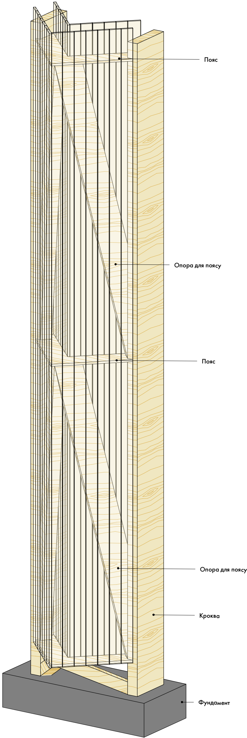
Конструктивна схема оболонки, загальний вид
