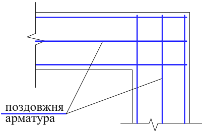
Деталь стиковки арматури в кутах монолітних фундаментів
