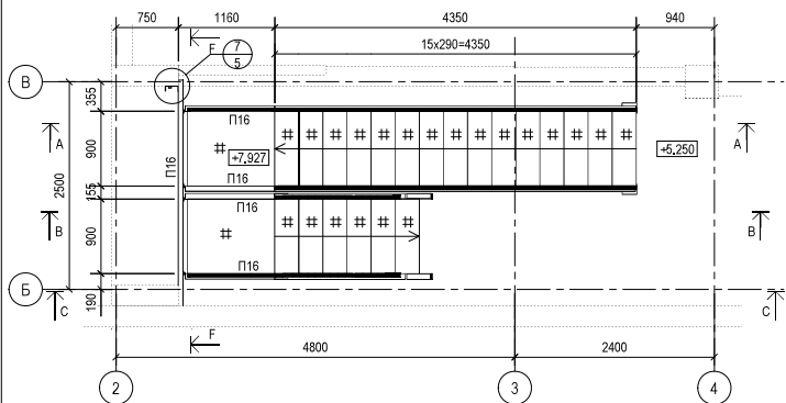
Схема розташування сходів в осях 2-4хБ-В
