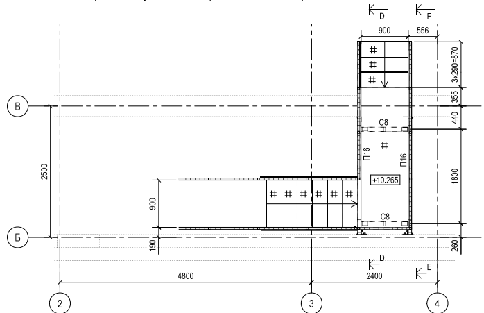
Схема розташування перехідної площадки на відм. +10.265
