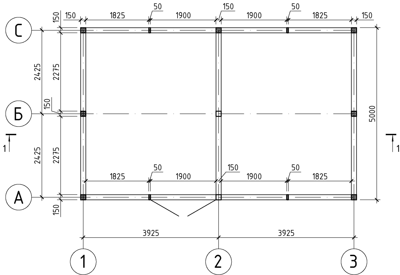
План каркаса
