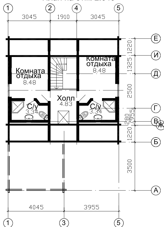
План на отм. 2.640
