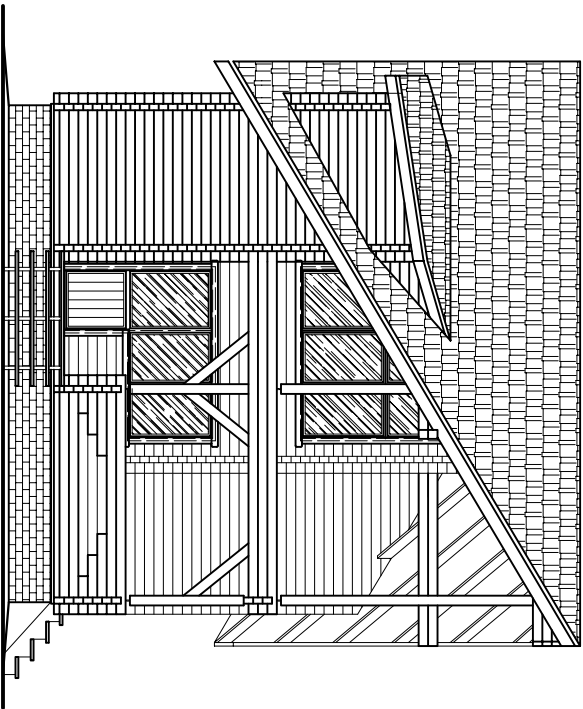
ФАСАД В ОСЯХ 6-1
