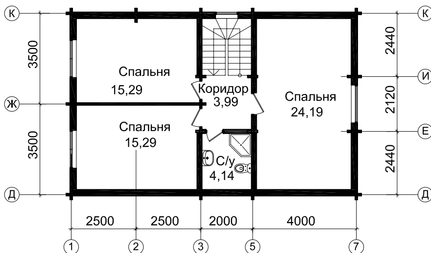
План на отм. 3,132
