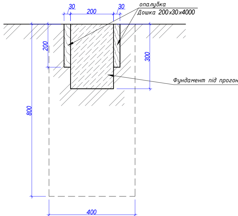
Розріз 1-1 М1:10
