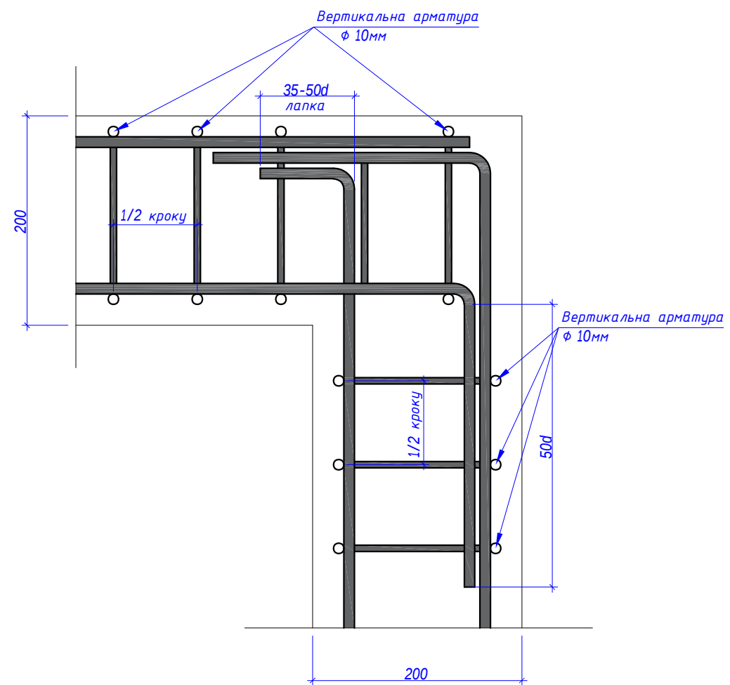
Вузол Б М1:5
