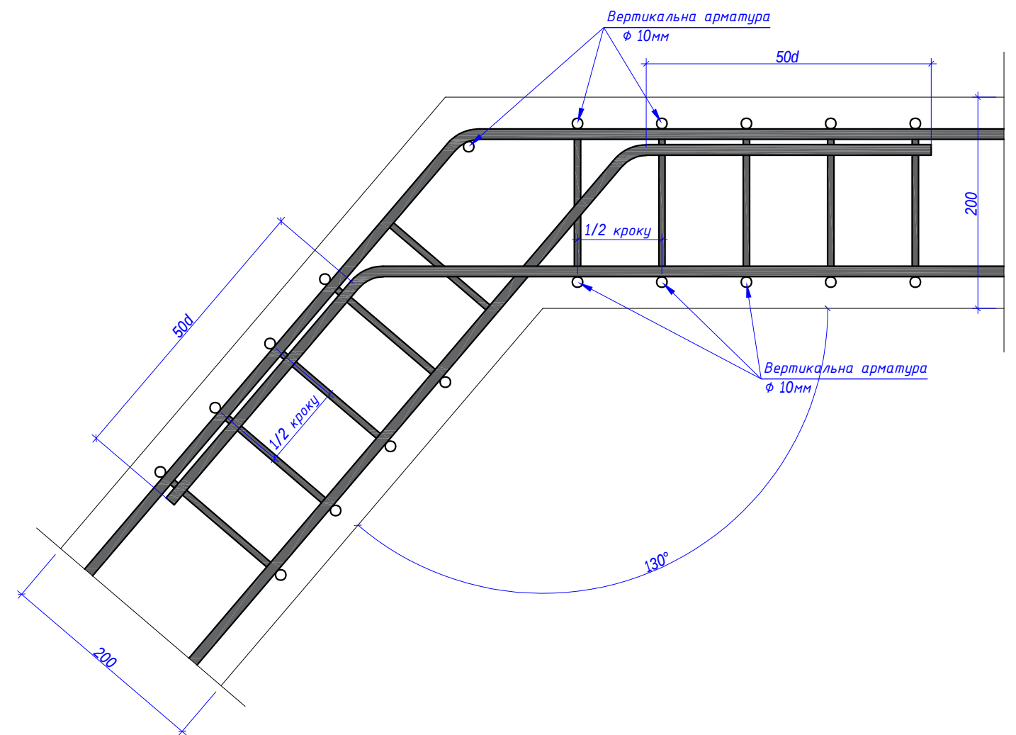
Вузол В М1:5
