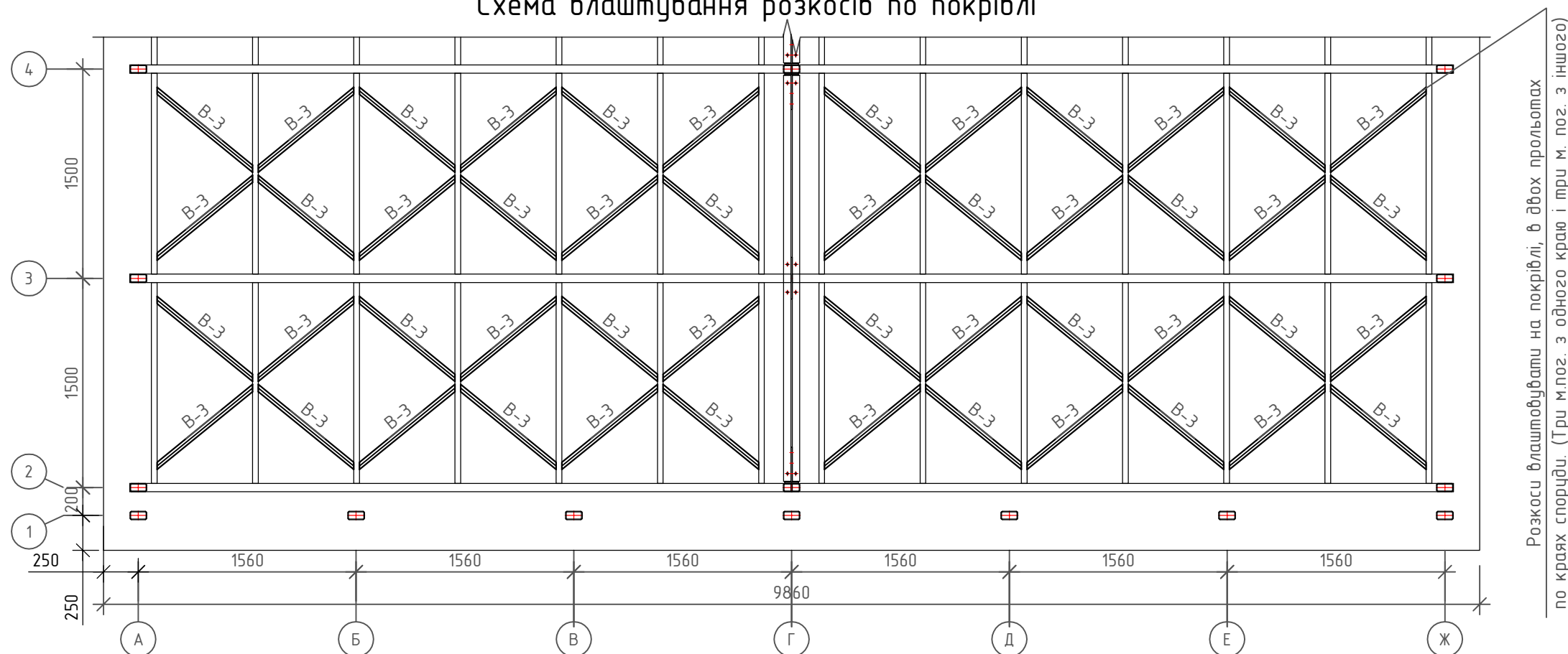
Схема влаштування розкосів по покрівлі
