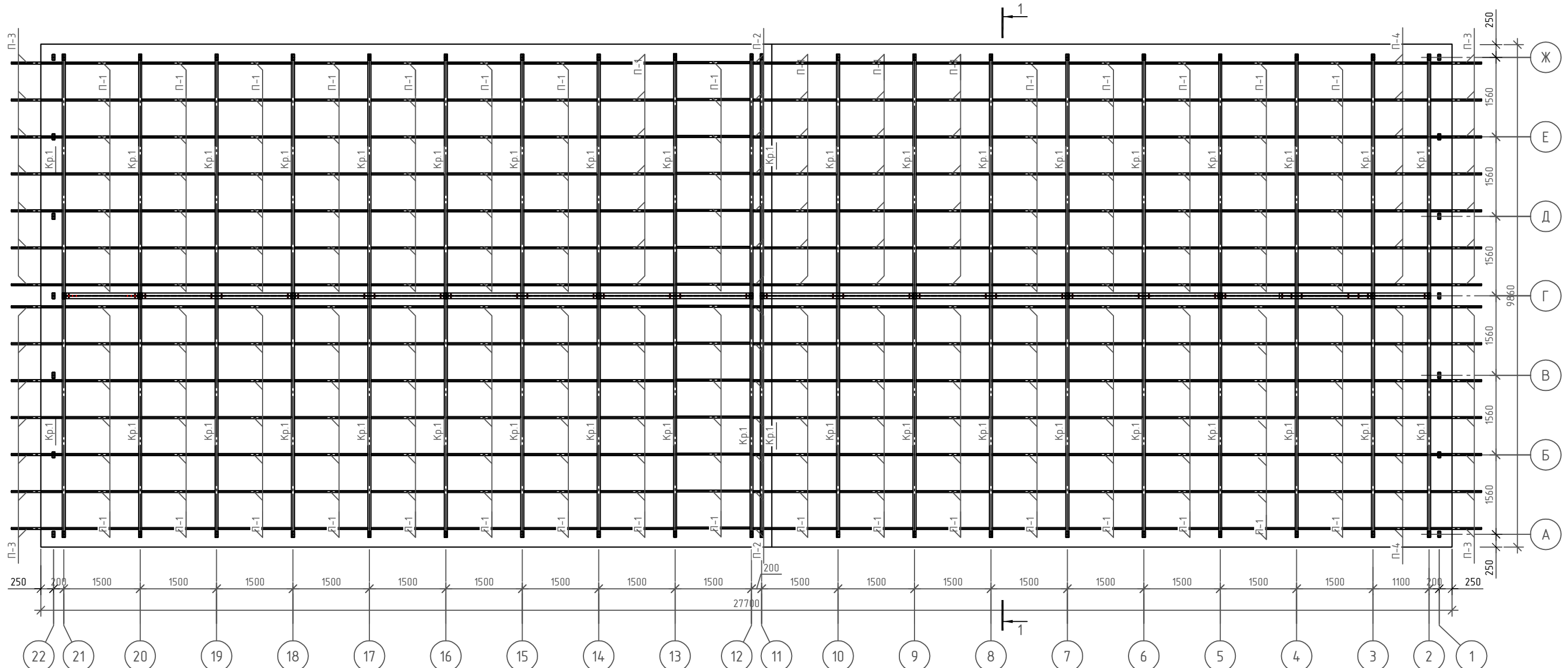
Схема розташування кроків і прогонів
