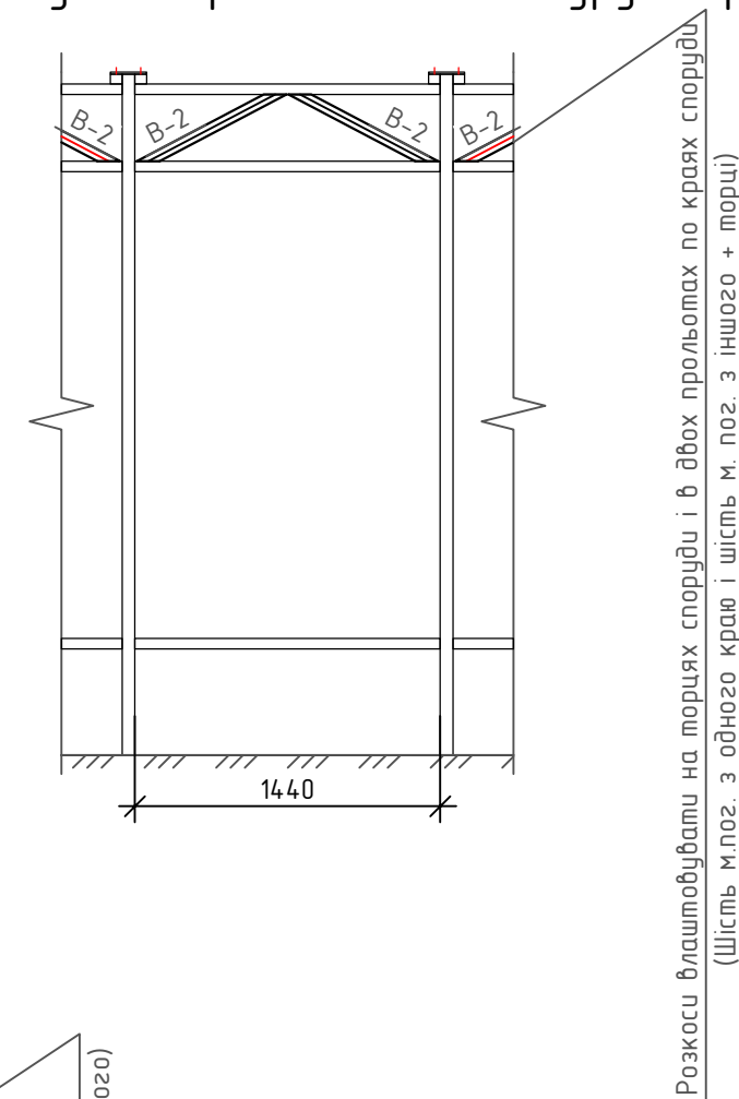
Схема влаштування розкосів по контуру споруди
