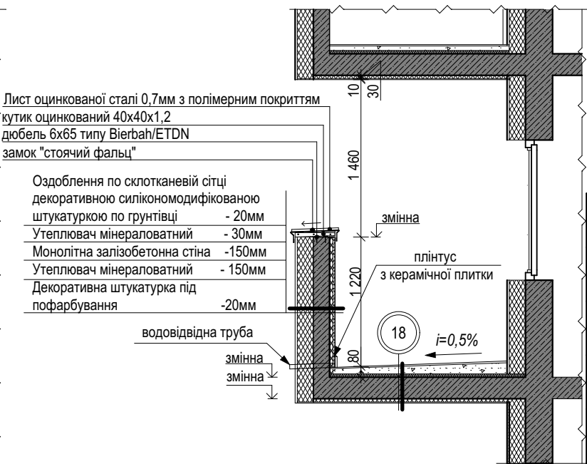
Типовий розріз 2-2
