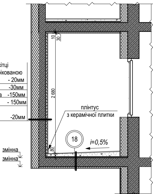
Типовий розріз 1-1
