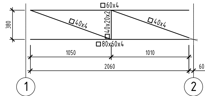
Геометрична схема ферми Ф-7 (1 од.) перерізи
