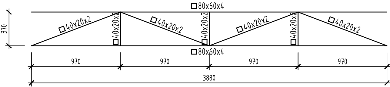
Геометрична схема ферми Ф-5 (1 од.) перерізи
