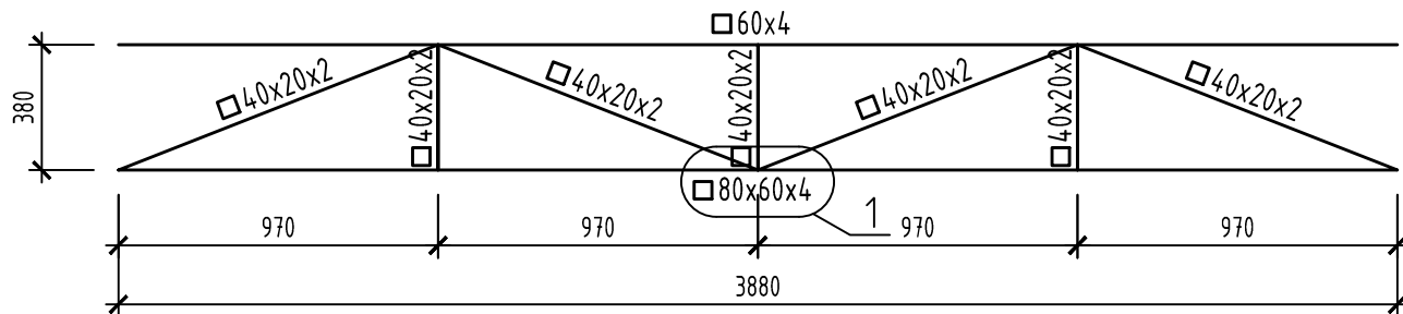
Геометрична схема ферми Ф-6 (1 од.) перерізи
