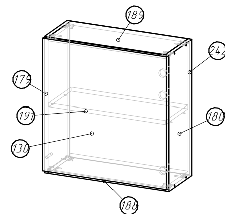
3_Шафа_588_232_617
