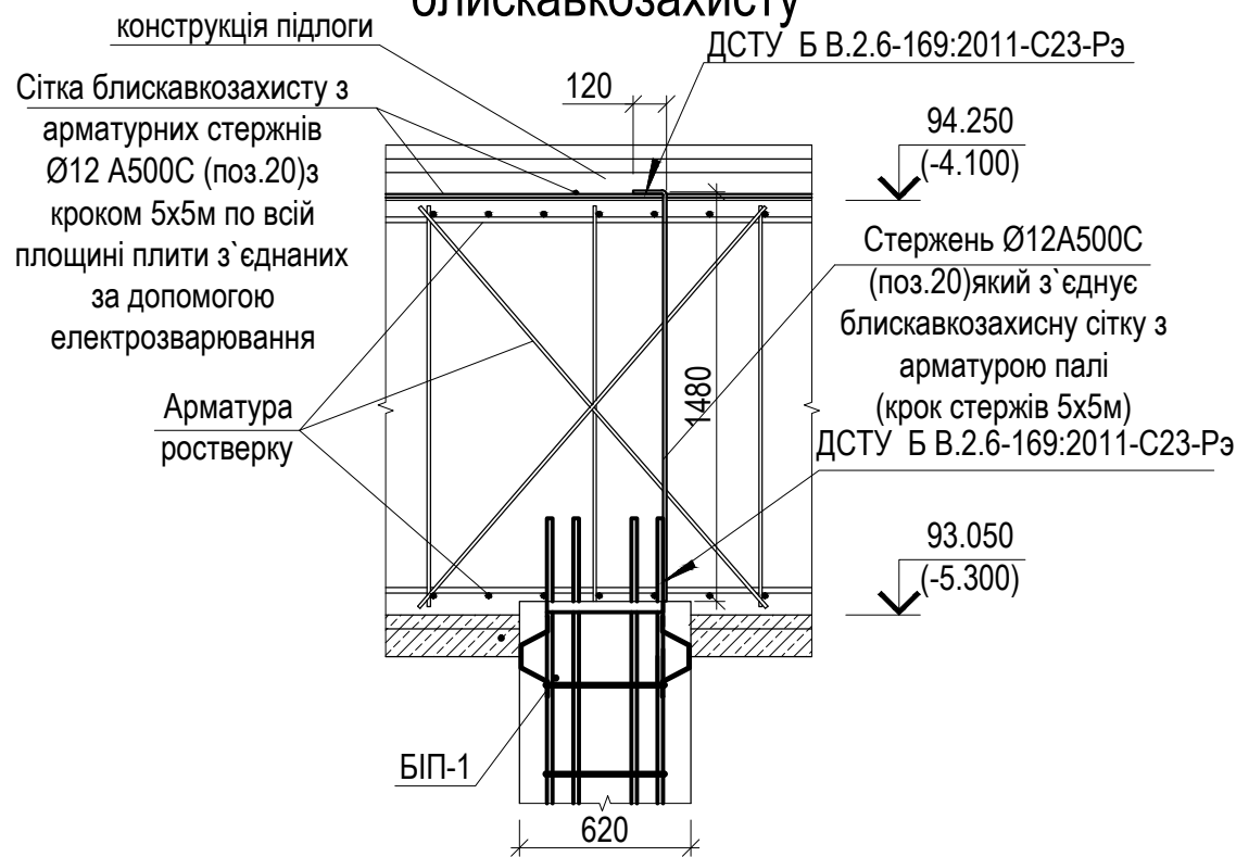
Вузол з'єднання елементів блискавкозахисту
