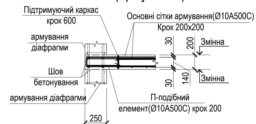
1 - 1(армування)
