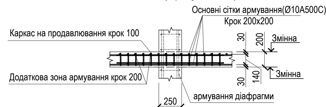
2 - 2 (армування)
