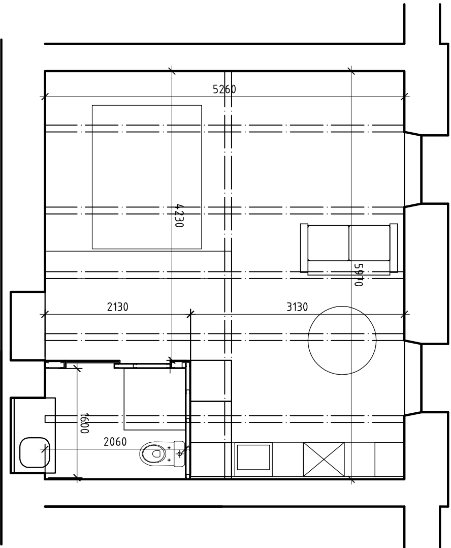
Проектований план приміщення (для довідки)
