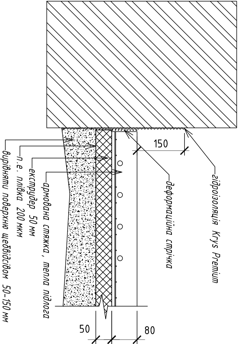
Деталь підлоги
