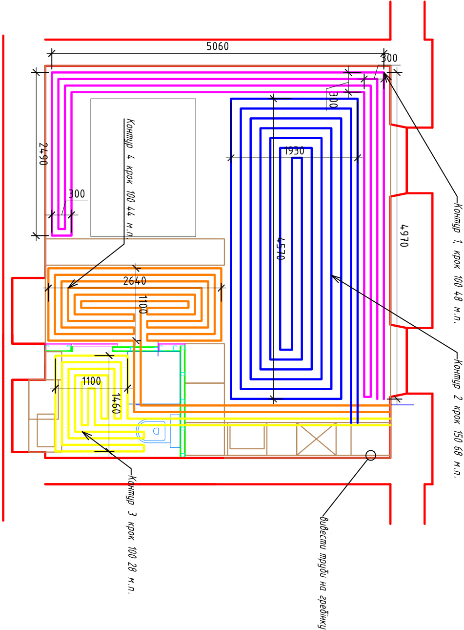
Схема виконання робіт по теплій підлозі
