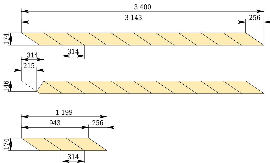
Чертеж тетивы
