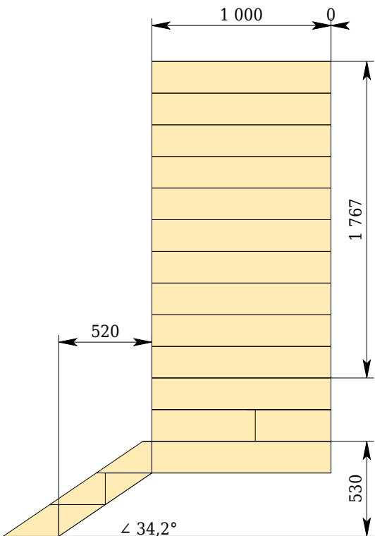
Вид спереди
