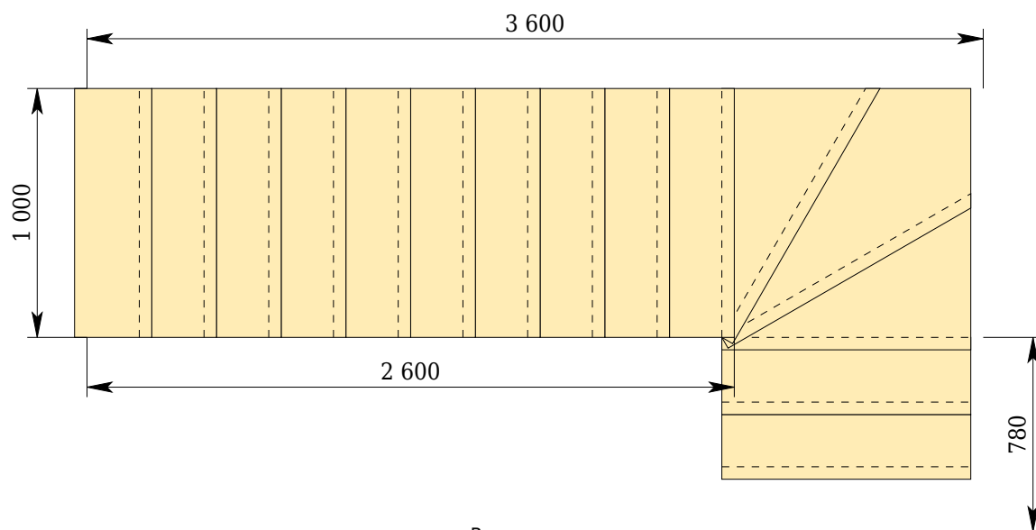
Вид сверху
