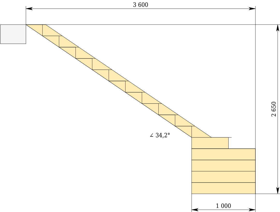
Вид сбоку
