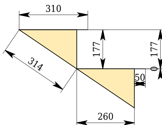
Чертеж шаблона ступеней
