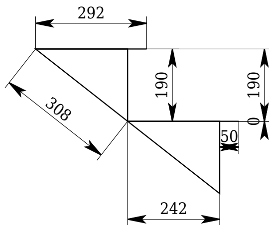
Креслення шаблону сходів
