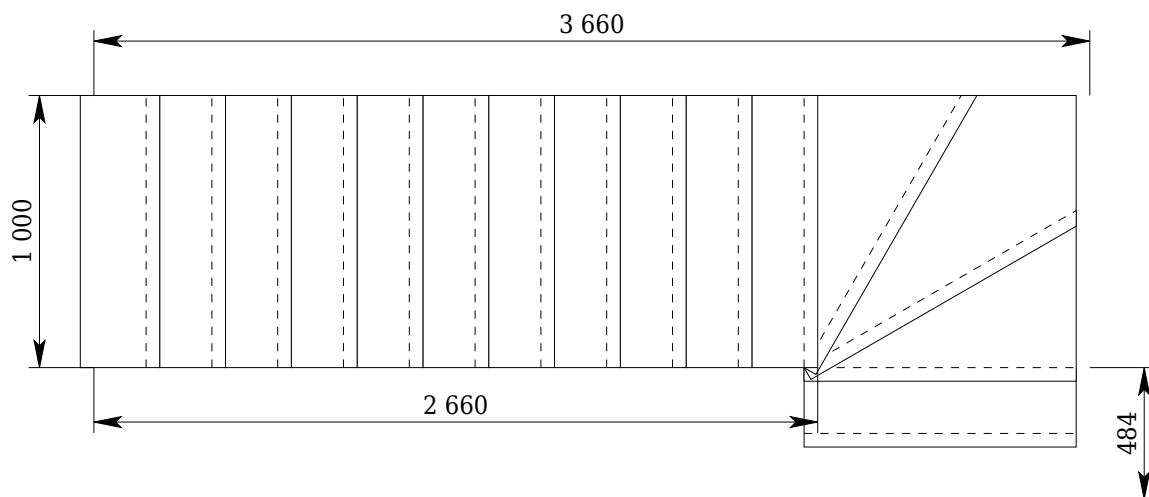
Вид сверху
