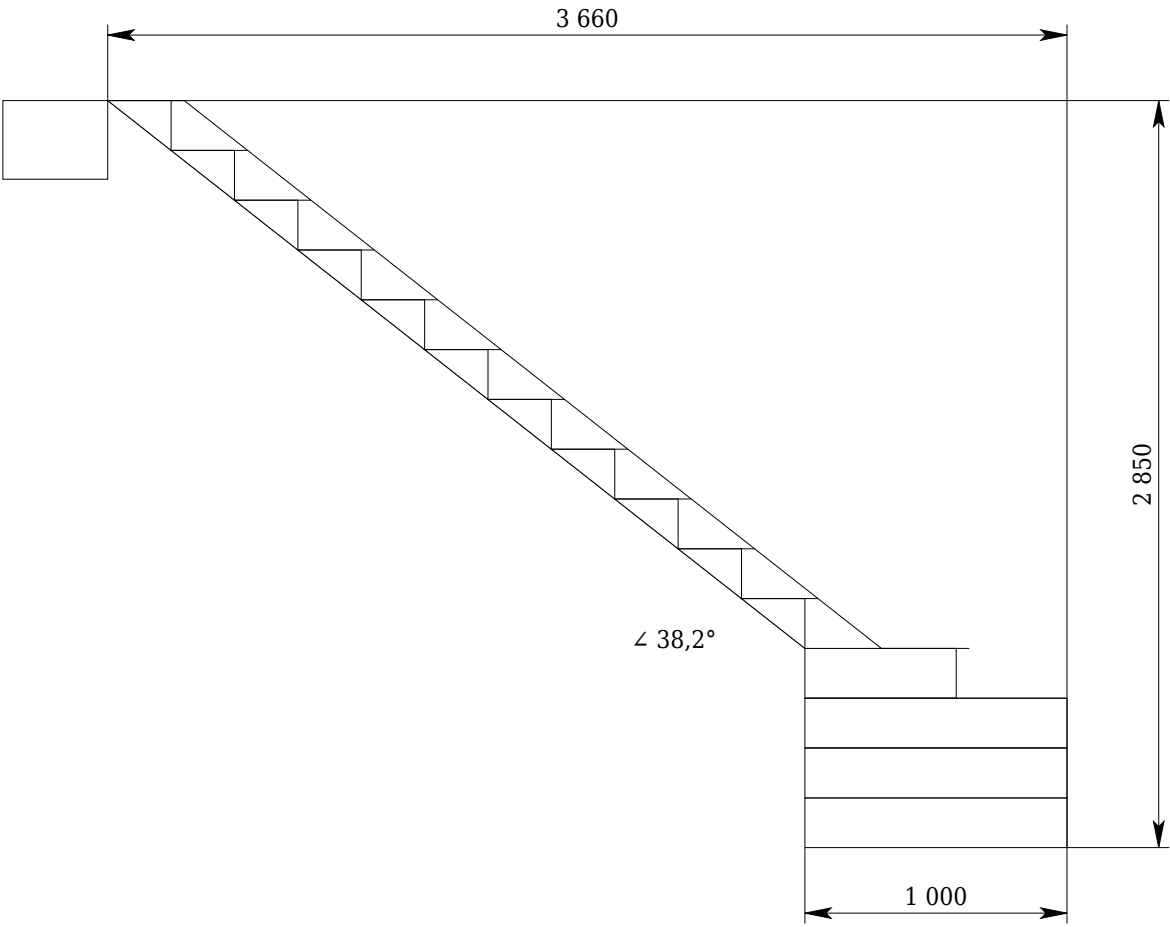
Вид збоку
