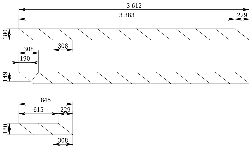
Креслення тятиви
