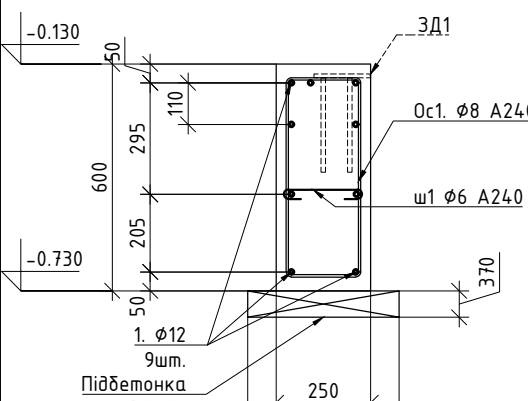
2-2 ФБ1 Арматура
