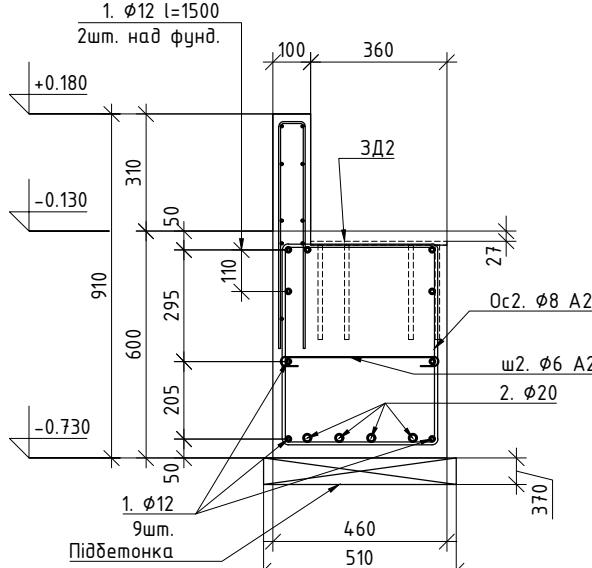
3-3 ФБ1 Арматура
