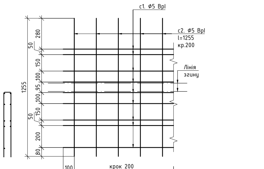
Сітка С1
