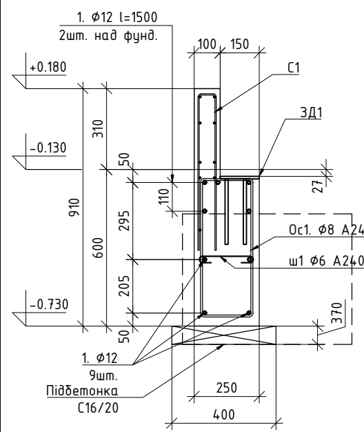
1-1 ФБ1 Арматура
