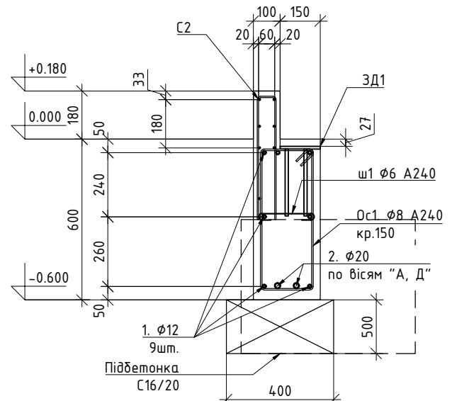
5-5 ФБ2 Арматура
