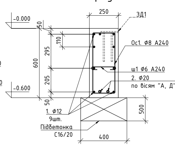
5-5 ФБ2 Арматура
