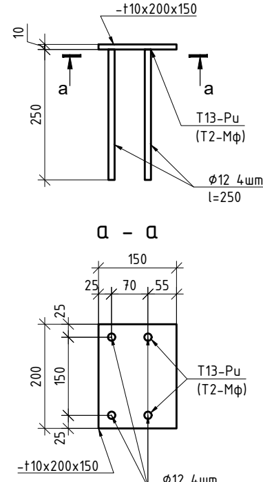
Закладна деталь ЗД1
