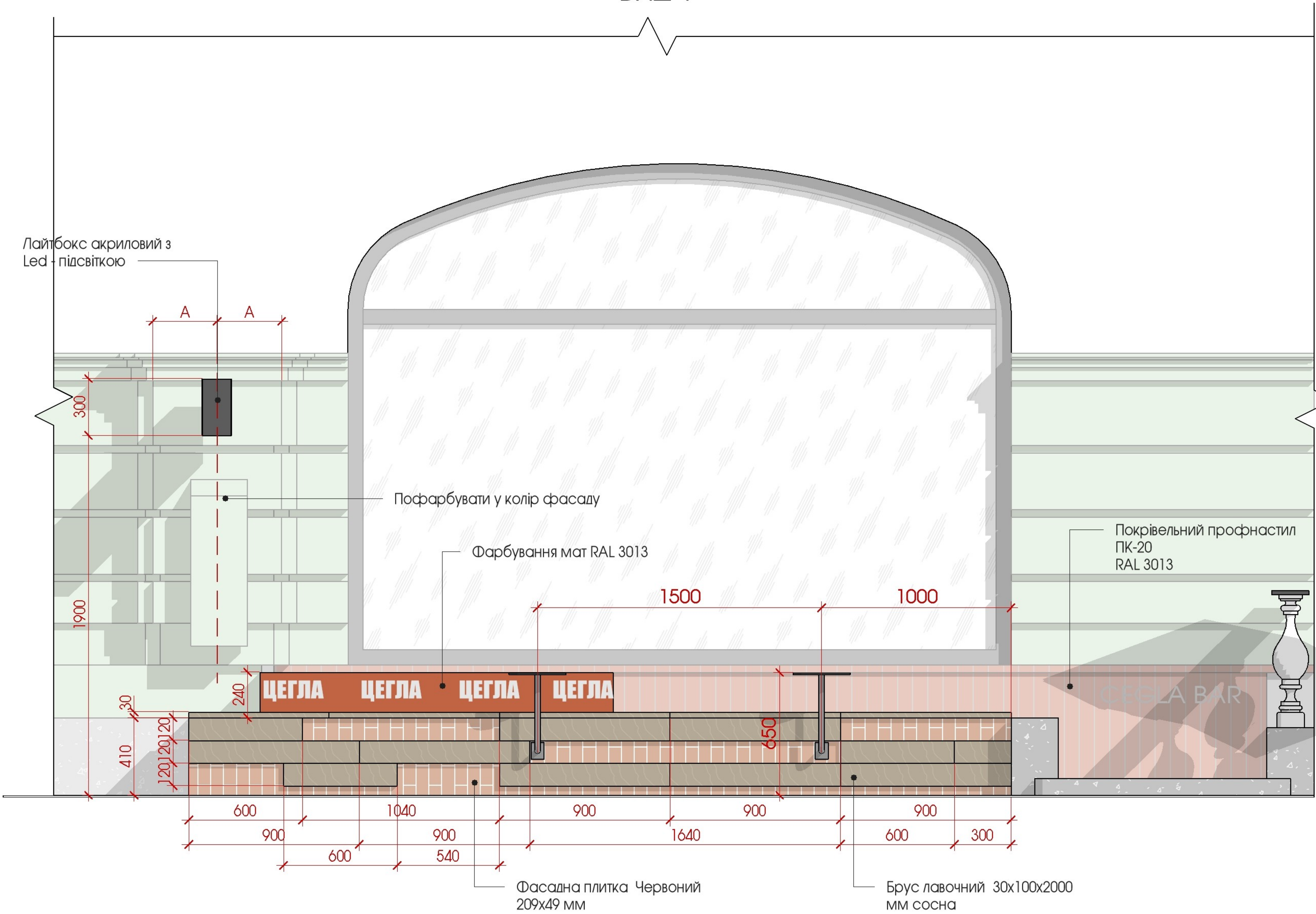
ВИД 1
