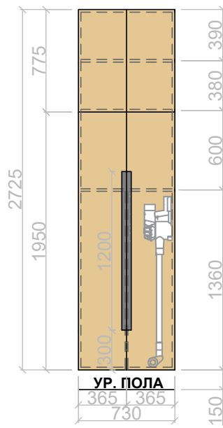
ХОЗ. ШКАФ
