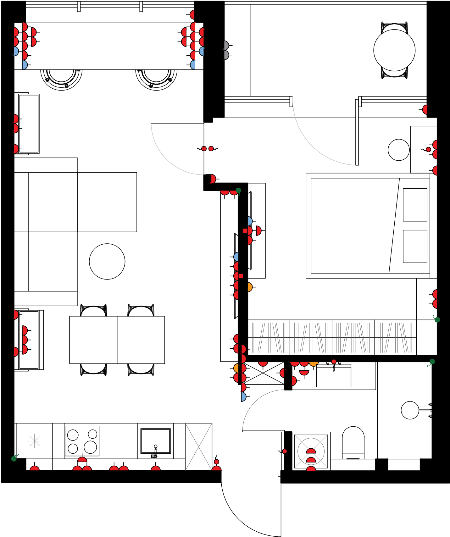
ПЛАН ЭЛЕКТРИЧЕСТВА С МЕБЕЛЬЮ 1:40
