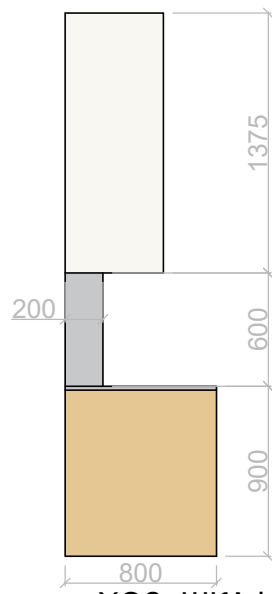
ХОЗ. ШКАФ
