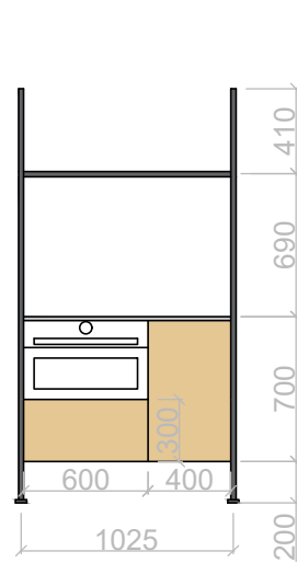
БАР-СТЕЛЛАЖ
