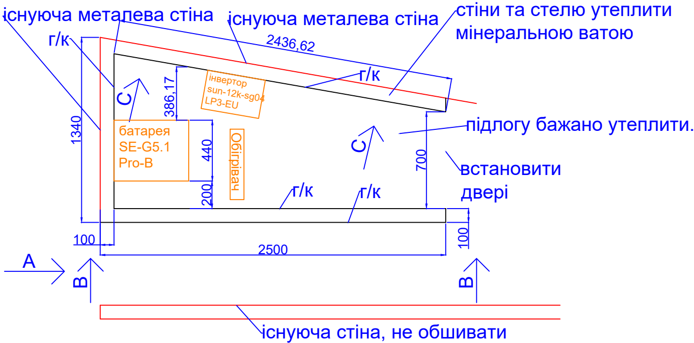
ВИД ЗВЕРХУ
