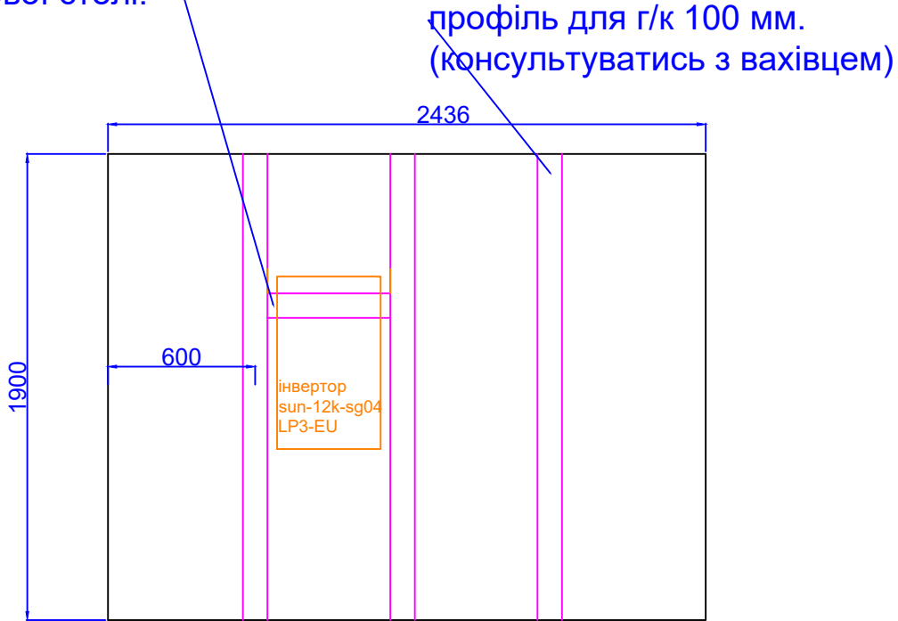
ВИД С-С
