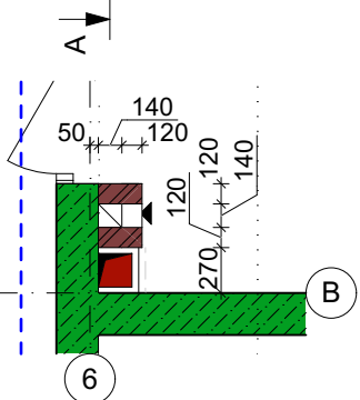
План 1-го поверху М 1:50
