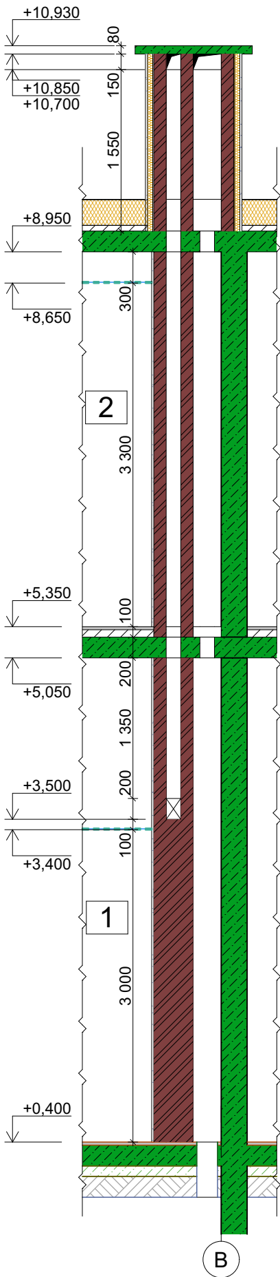
Січення А-А М 1:50
