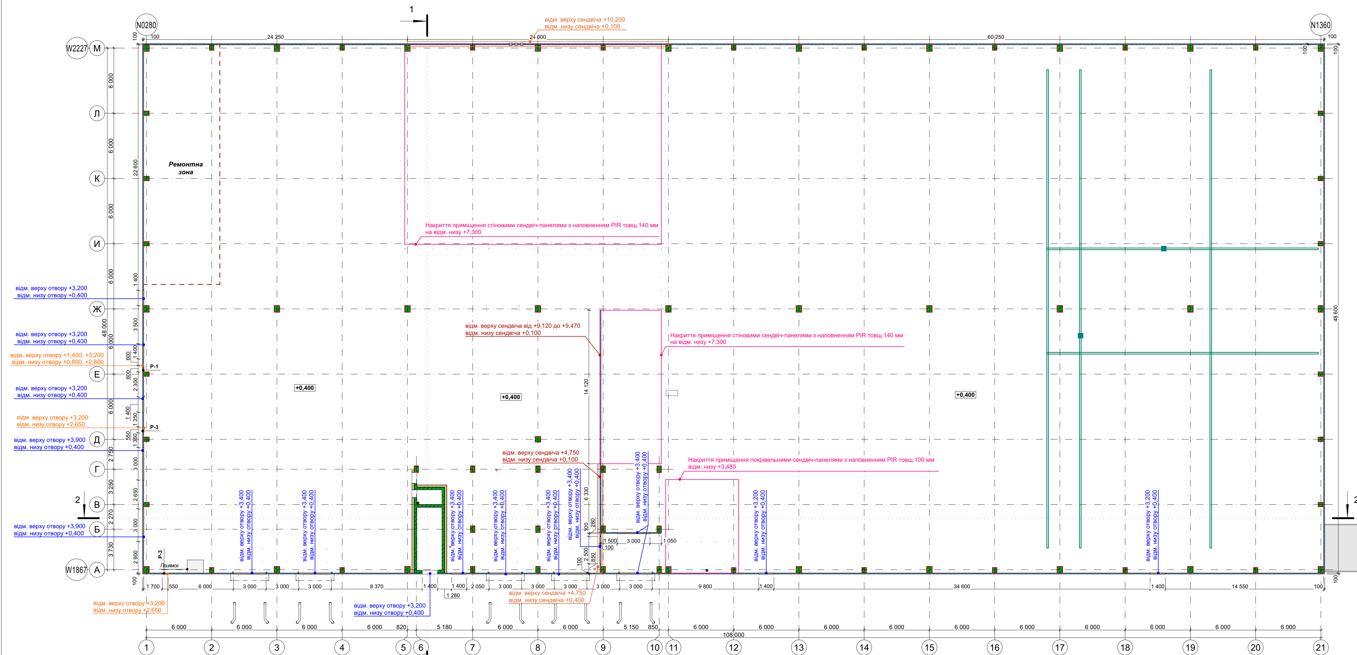
Розбивочний план 1-го поверху. М 1:200
