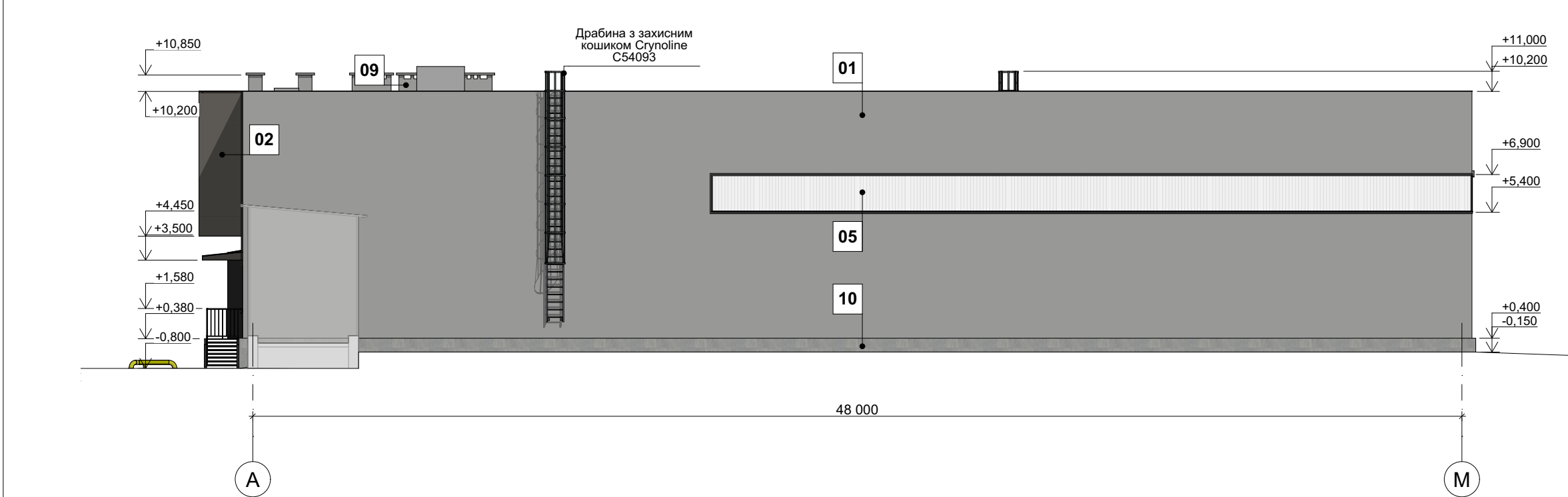
Фасад в осях А-М. М 1:200
