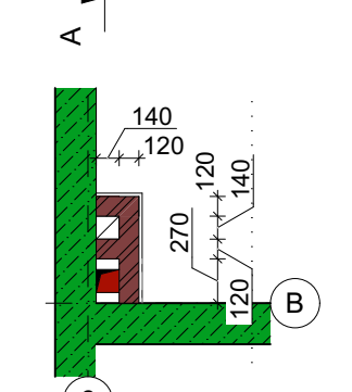
План 2-го поверху М 1:50
