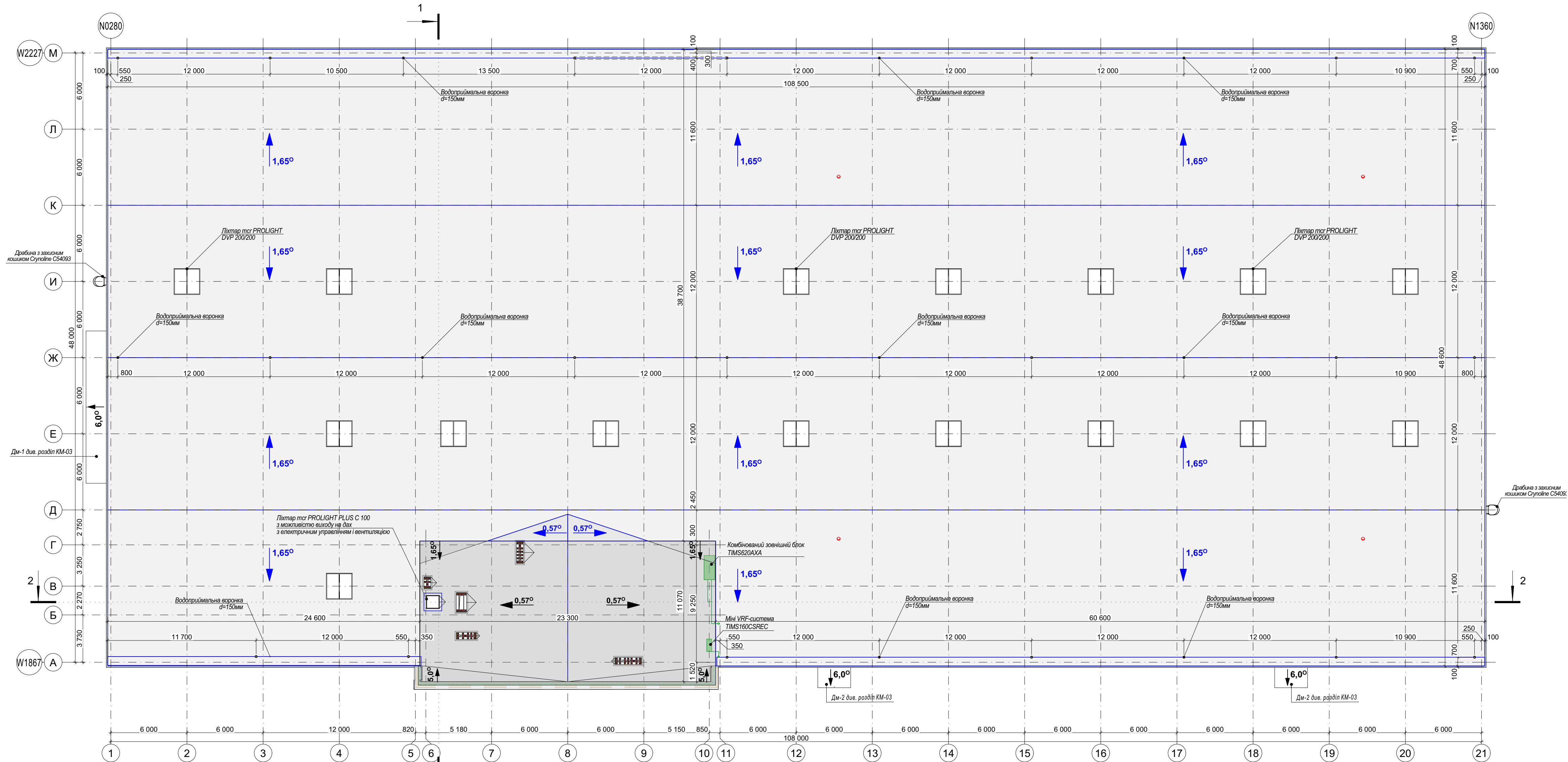
План покрівлі. М 1:200
