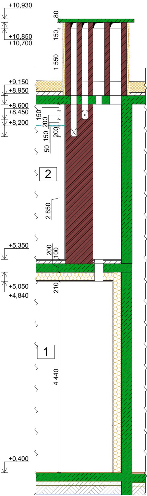
Січення Б-Б М 1:50
