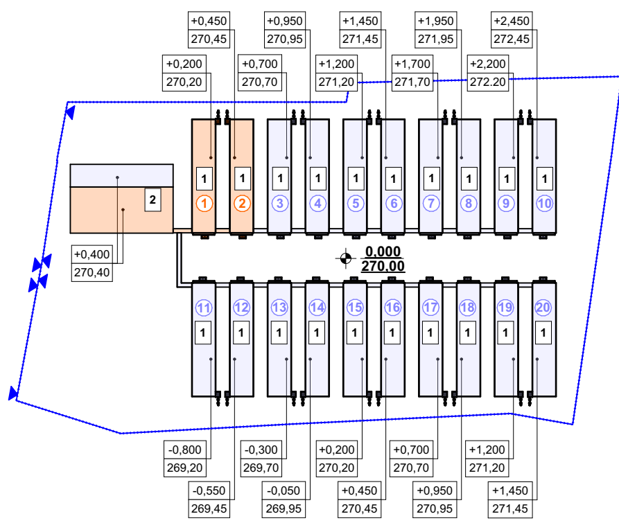
План-схема
