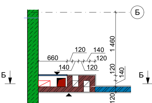
План 2-го поверху М 1:50
