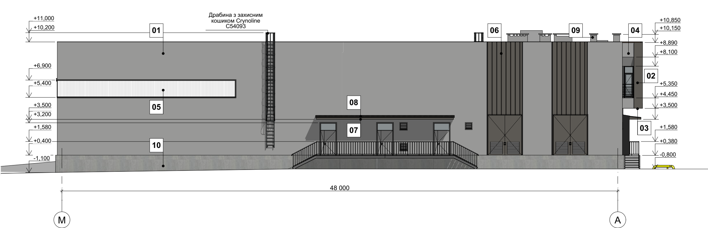
Фасад в осях М-А. М 1:200
