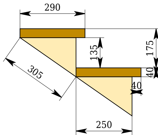
Чертеж шаблона ступеней
