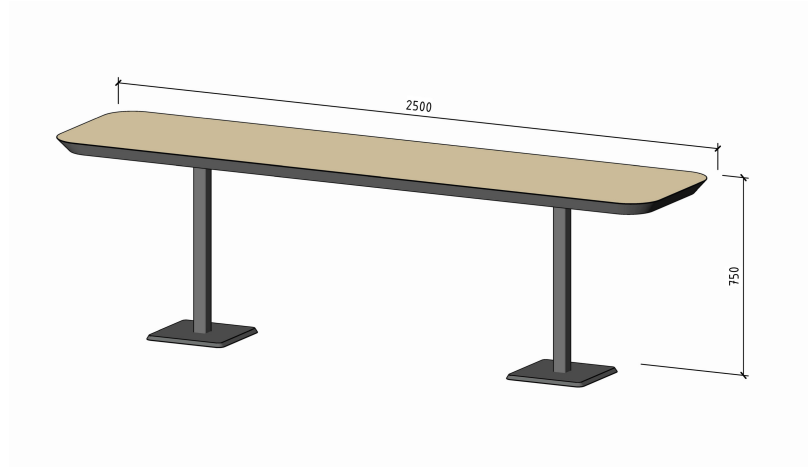
Стіл для нарад під індивідуальне замовлення (МБ-02). 3D-схема
