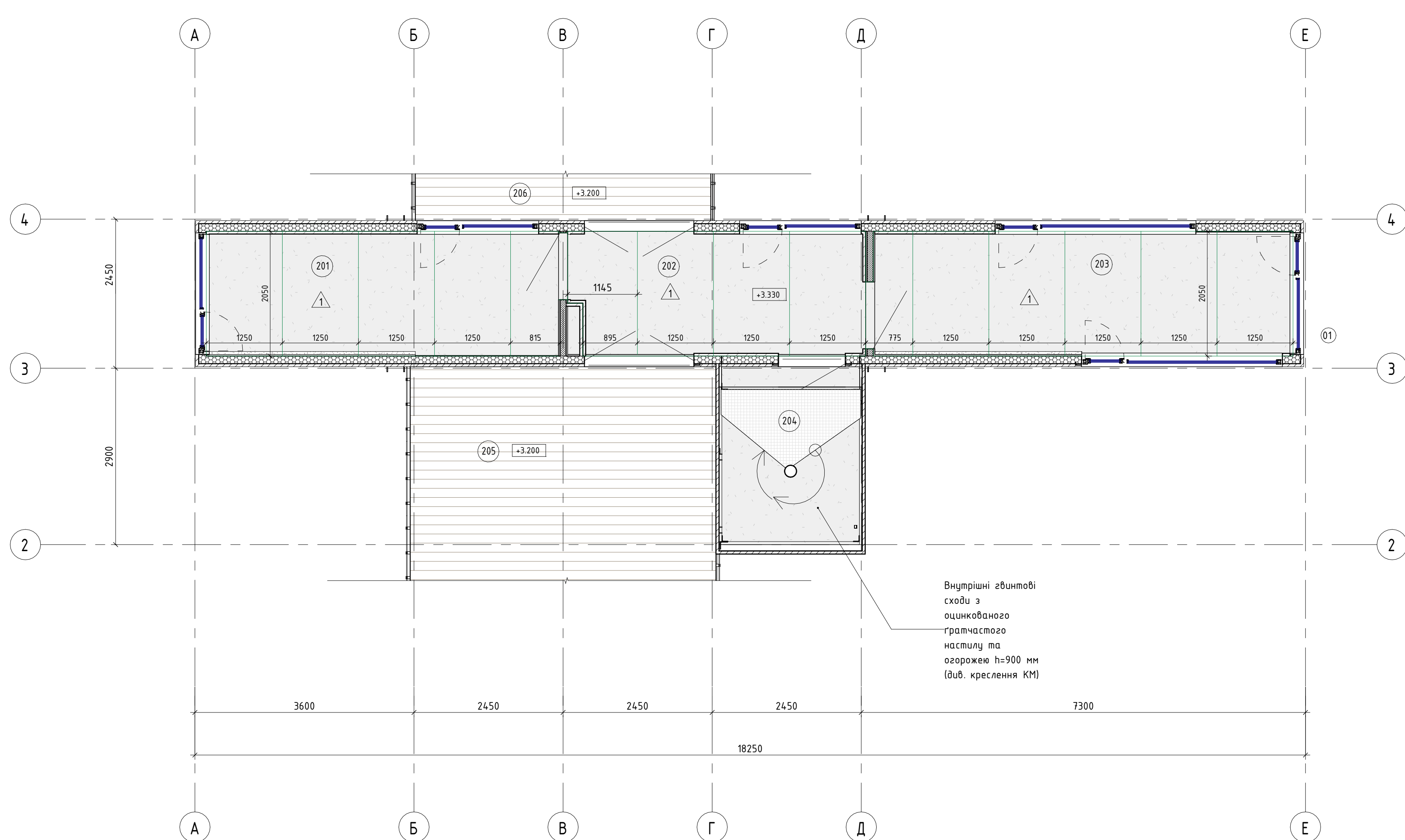
План підлог 2-го поверху на відм. +3,330 М 1 : 50
