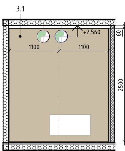
Розгортка 4.3 М 1 : 50
