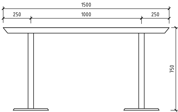
Стіл для нарад під індивідуальне замовлення (МБ-02.1). Вид спереду М 1:20
