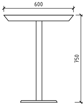
Стіл для нарад під індивідуальне замовлення (МБ-02). Вид збоку М 1:20
