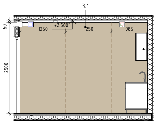
Розгортка 3.3 М 1 : 50
