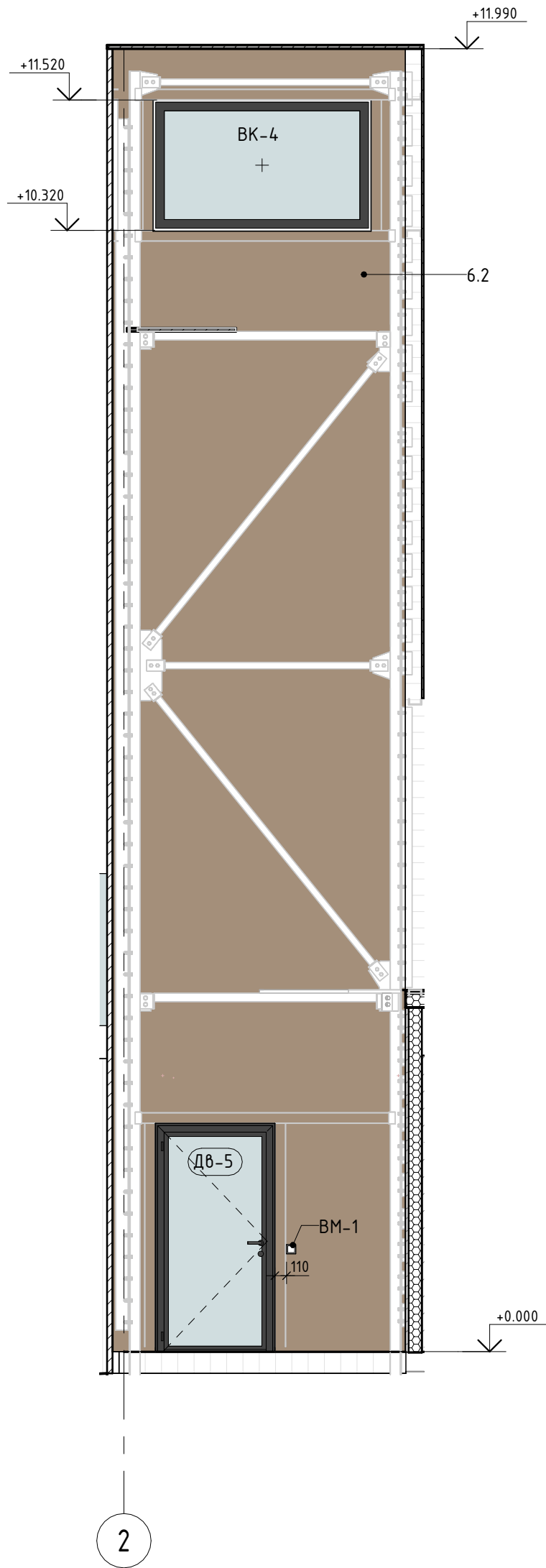
Розгортка 10.1 М 1 : 50
