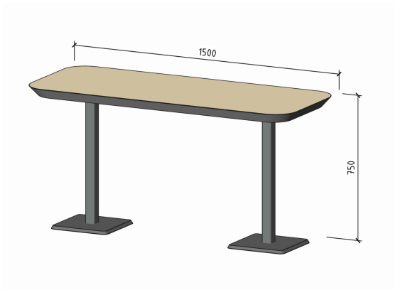
Стіл для нарад під індивідуальне замовлення (МБ-02.1). 3D-схема
