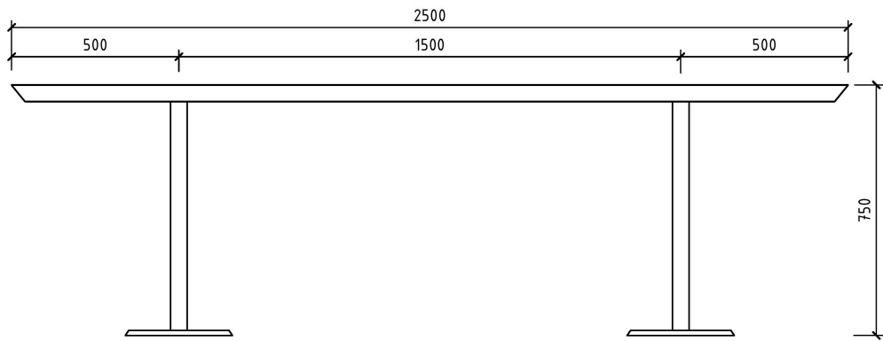
Стіл для нарад під індивідуальне замовлення (МБ-01). Вид спереду М 1:20
