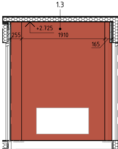
Розгортка 6.2 М 1 : 50
