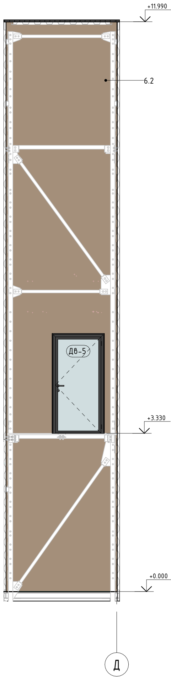
Розгортка 10.2 М 1 : 50
