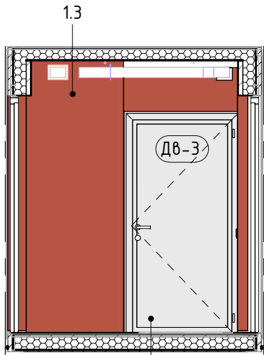
Розгортка 8.1
