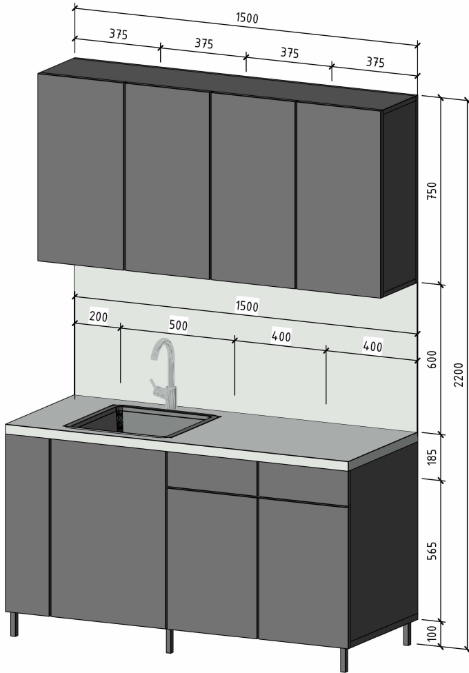
Кухонний блок під індивідуальне замовлення. 3D-схема
