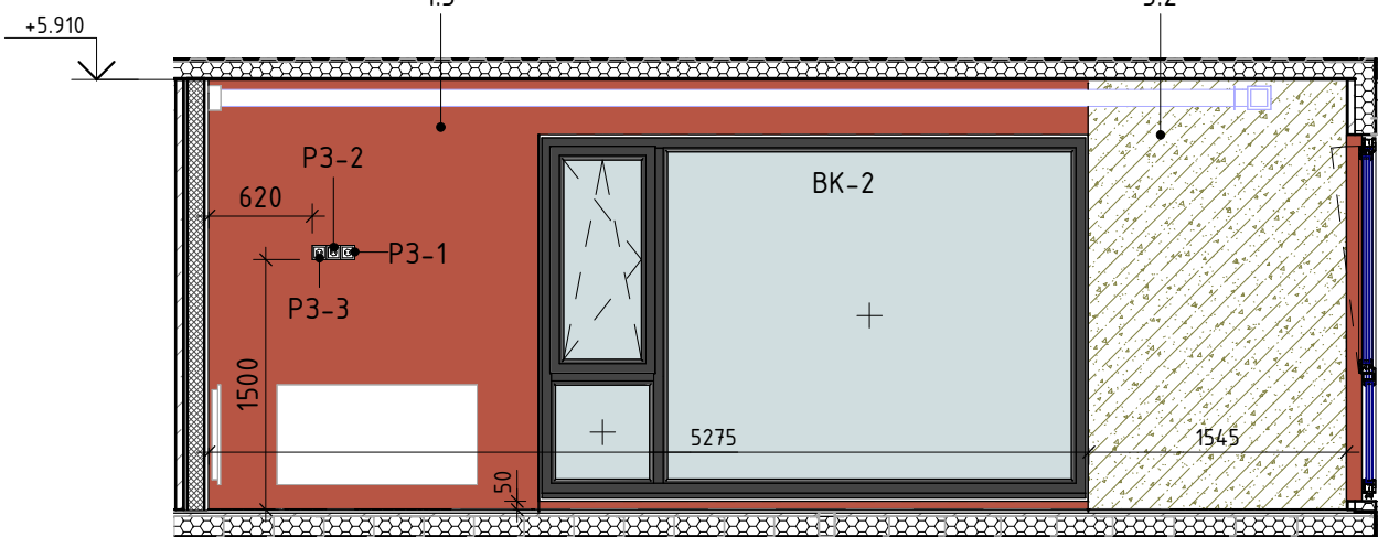
Розгортка 9.2
