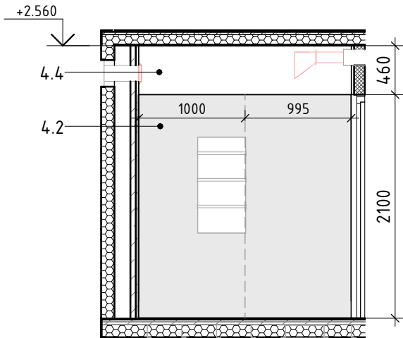
Розгортка 5.3 М 1 : 50
