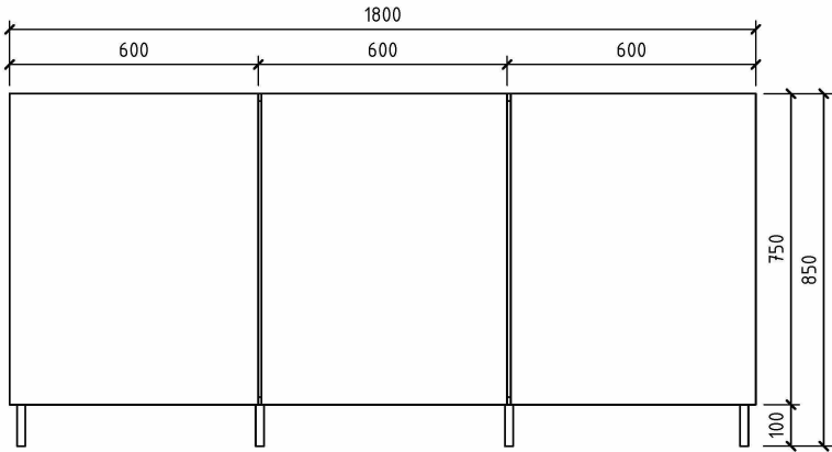
Комод під індивідуальне замовлення (МБ-05). Вид спереду М 1:20
