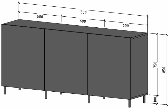
Комод під індивідуальне замовлення (МБ-05). 3D-схема
