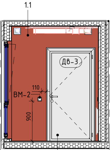
Розгортка 8.3
