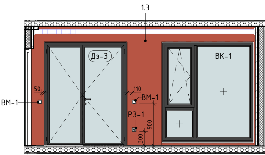
Розгортка 8.2
