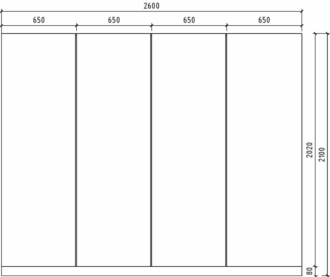
Шафа під індивідуальне замовлення (МБ-06). Вид спереду М 1:20
