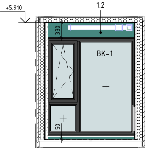
Розгортка 7.1
