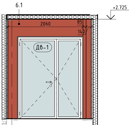
Розгортка 6.1 М 1 : 50
