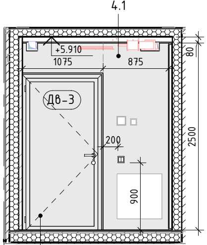
Розгортка 7.3
