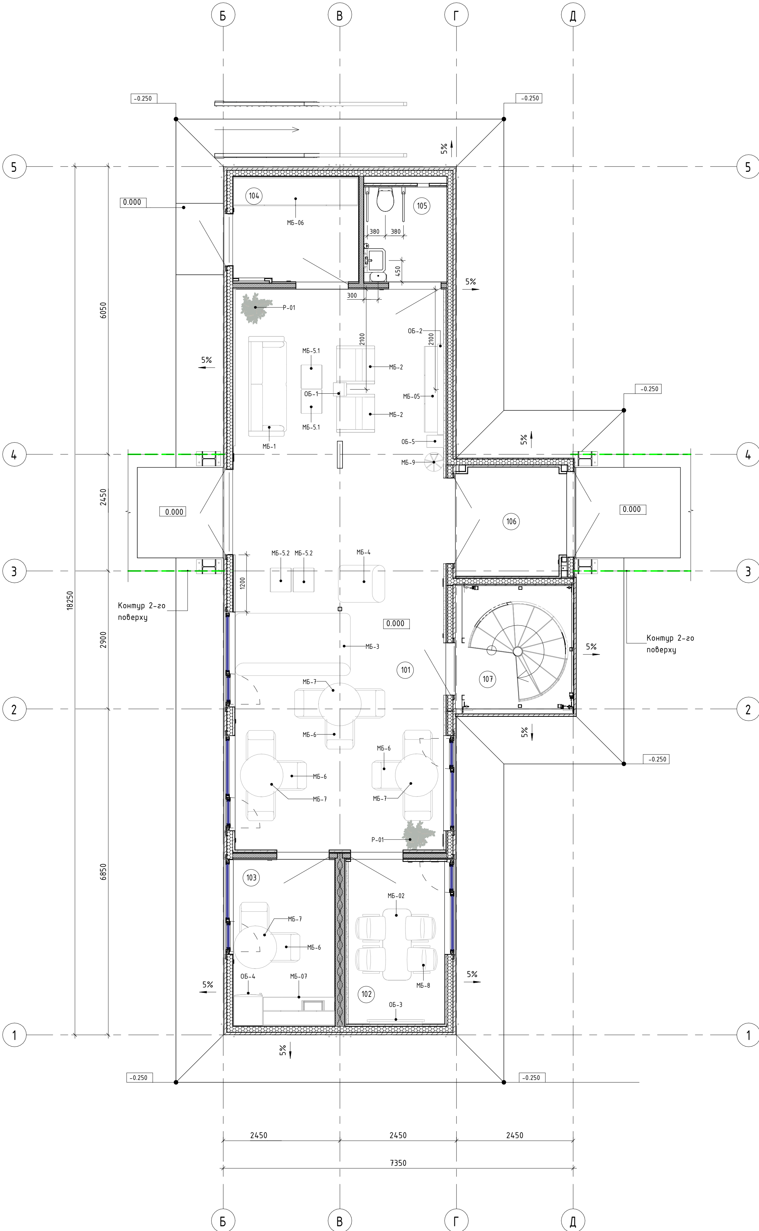
План цмеблювання 1-го поверху
