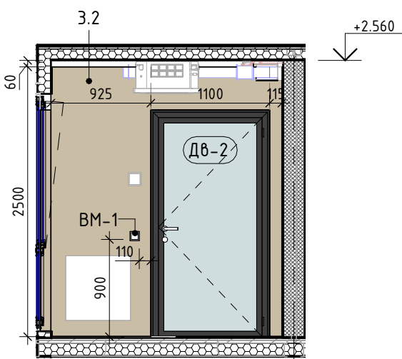
Розгортка 3.2 М 1 : 50
