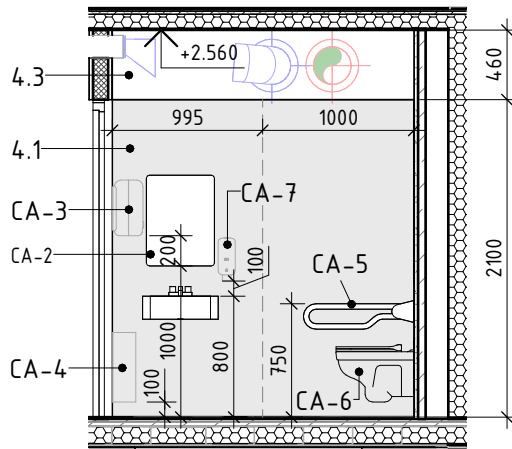
Розгортка 5.1 М 1 : 50
