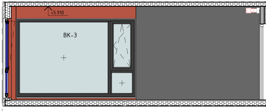
Розгортка 9.4
