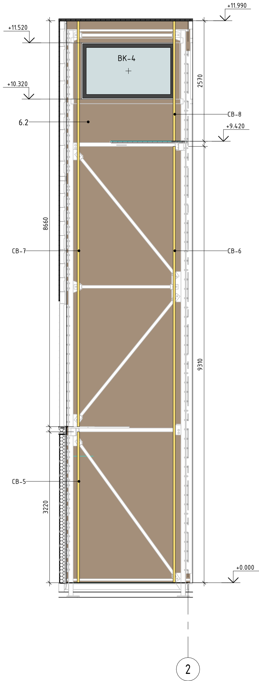
Розгортка 10.3 М 1 : 50
