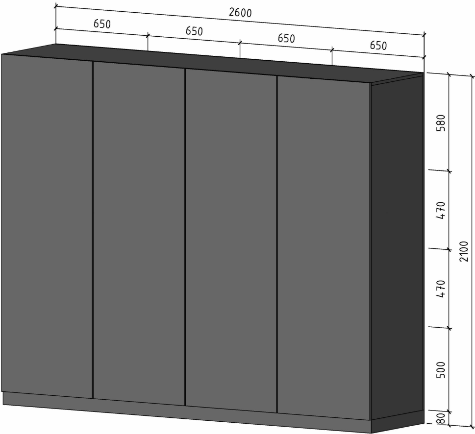
Шафа під індивідуальне замовлення (МБ-06). 3D-схема
