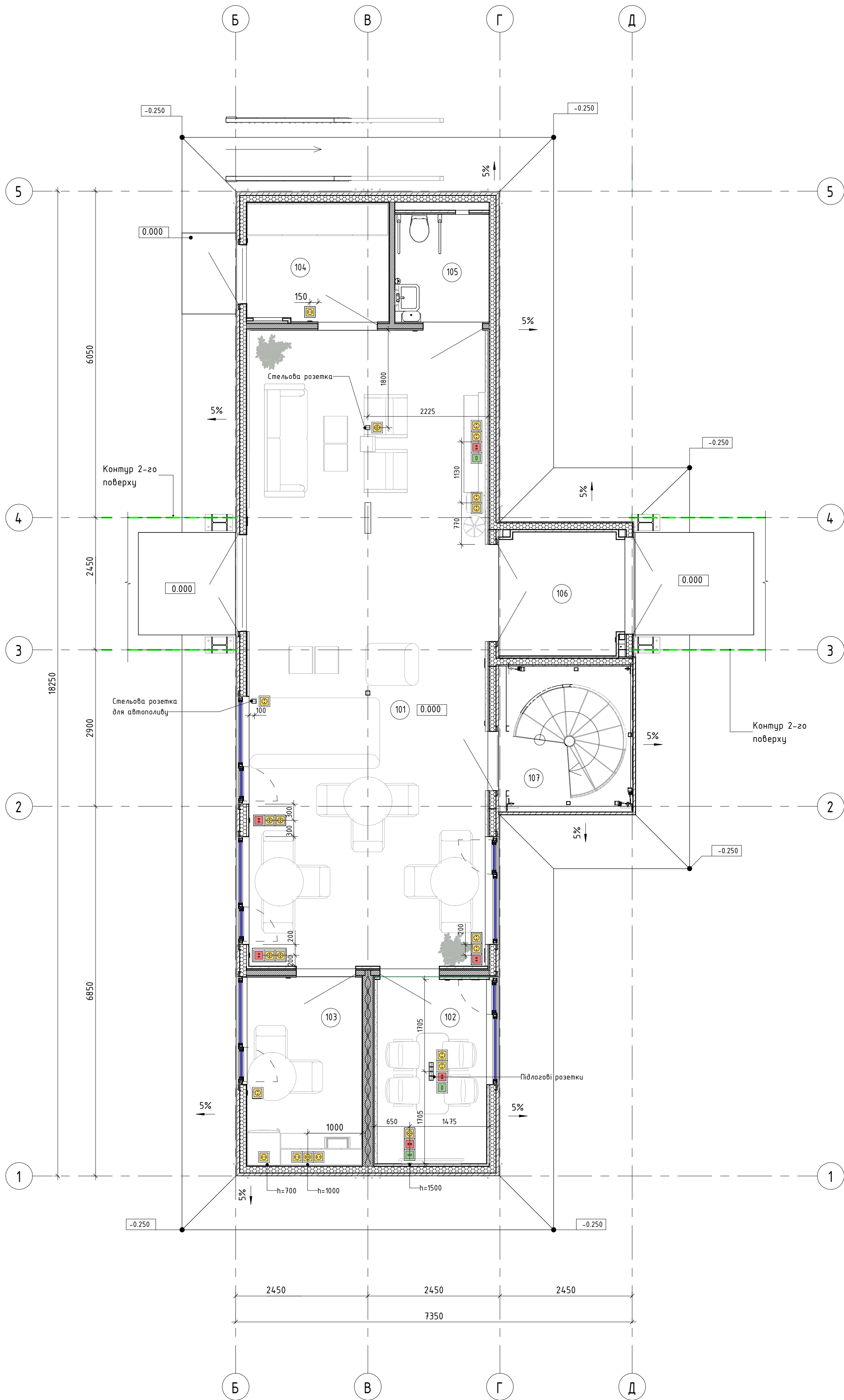
Схема влаштування розеток 1-го поверху М 1 : 50
