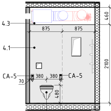
Розгортка 5.2 М 1 : 50
