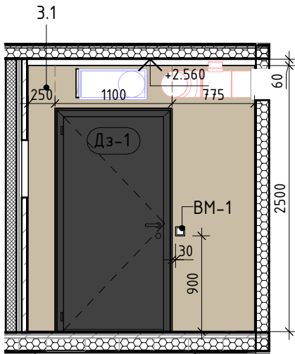
Розгортка 4.1 М 1 : 50
