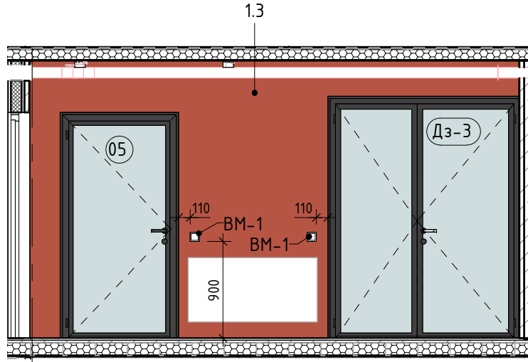
Розгортка 8.4
