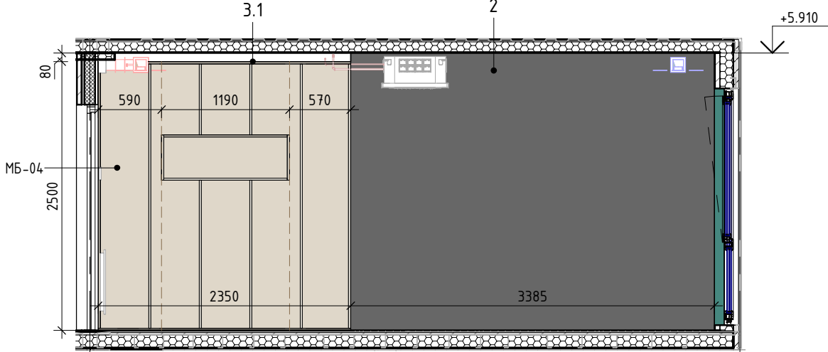
Розгортка 7.4
