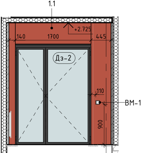
Розгортка 6.3 М 1 : 50
