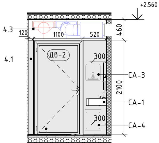
Розгортка 5.4 М 1 : 50
