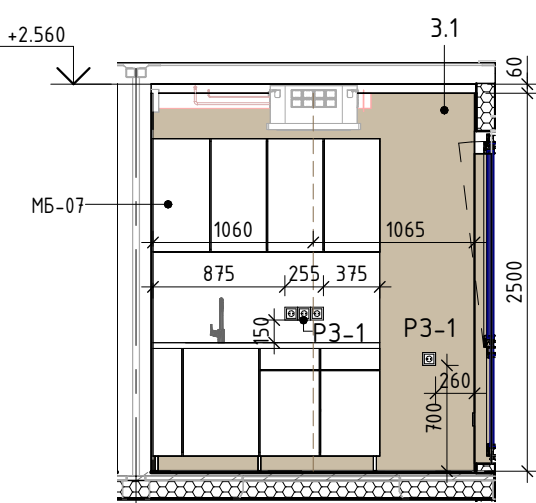
Розгортка 3.4 М 1 : 50
