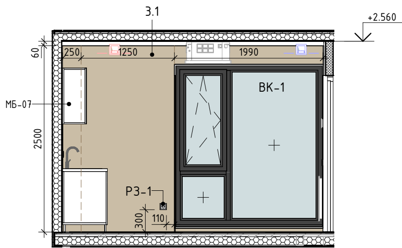
Розгортка 3.1 М 1 : 50
