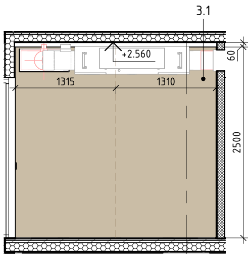
Розгортка 4.2 М 1 : 50
