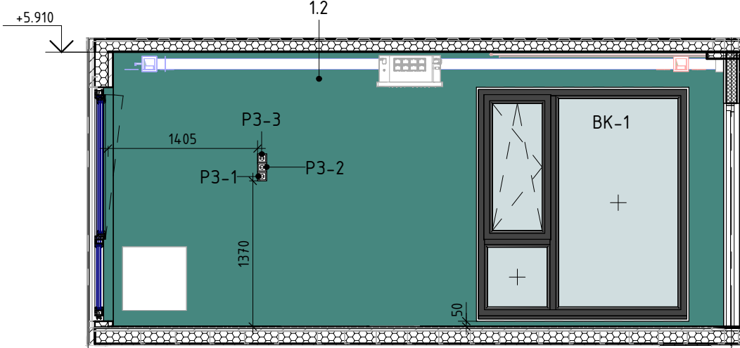
Розгортка 7.2
