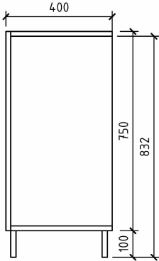
Комод під індивідуальне замовлення (МБ-05). Вид збоку М 1:20
