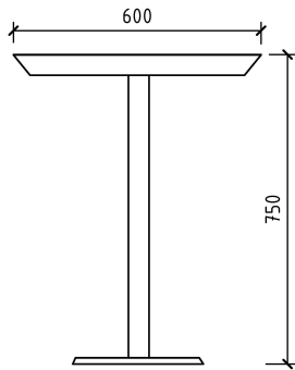
Стіл для нарад під індивідуальне замовлення (МБ-02.1). Вид збоку М 1:20
