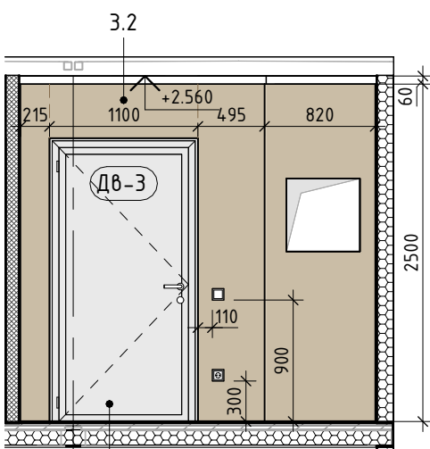
Розгортка 4.4 М 1 : 50
