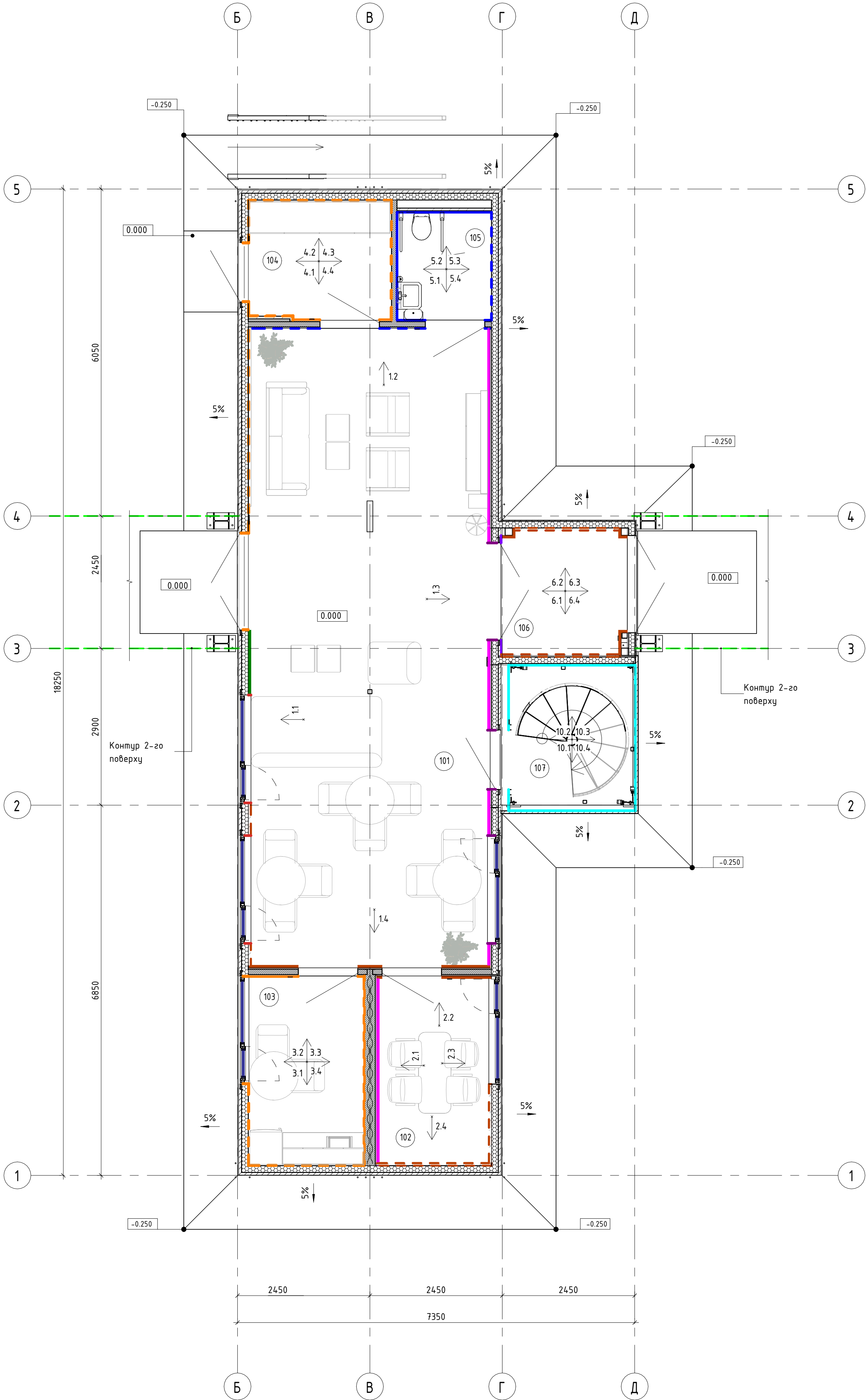
План розгортки і опорядження стін 1-го поверху М 1 : 50
