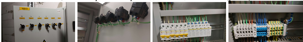
Рис. 6 – Щит освітлення ЩО
