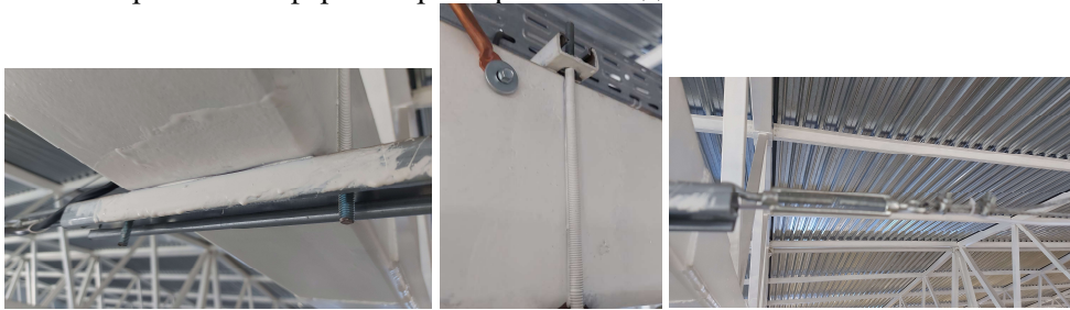
Рис. 3 – Кріплення тросу до ферм по осям 1, 6, 13, 20
