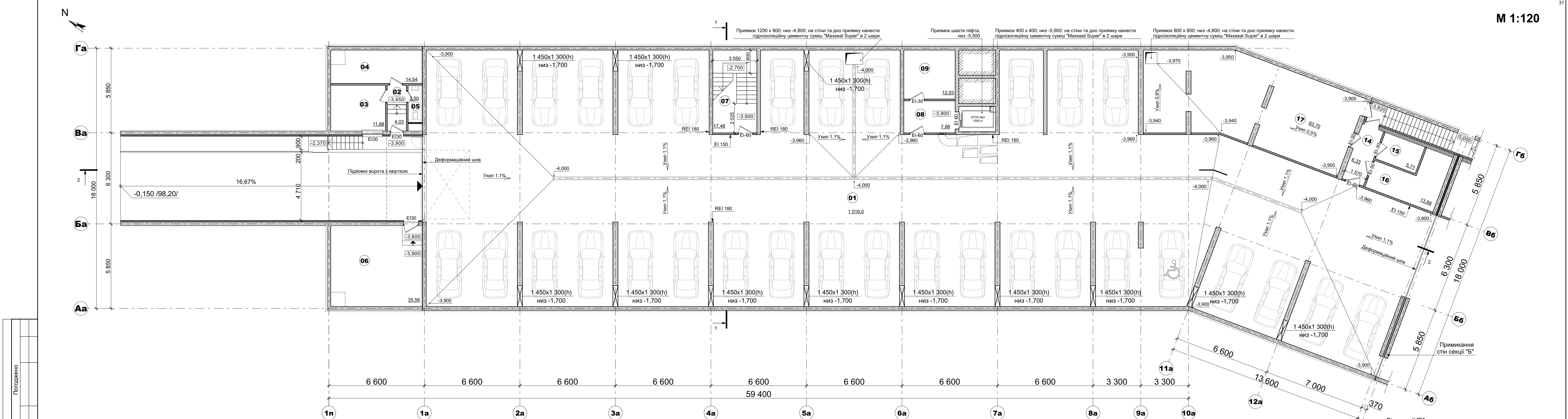
ЕКСПЛІКАЦІЯ ПРИМІЩЕНЬ ПІДВАЛУ (СЕКЦІЯ А)
