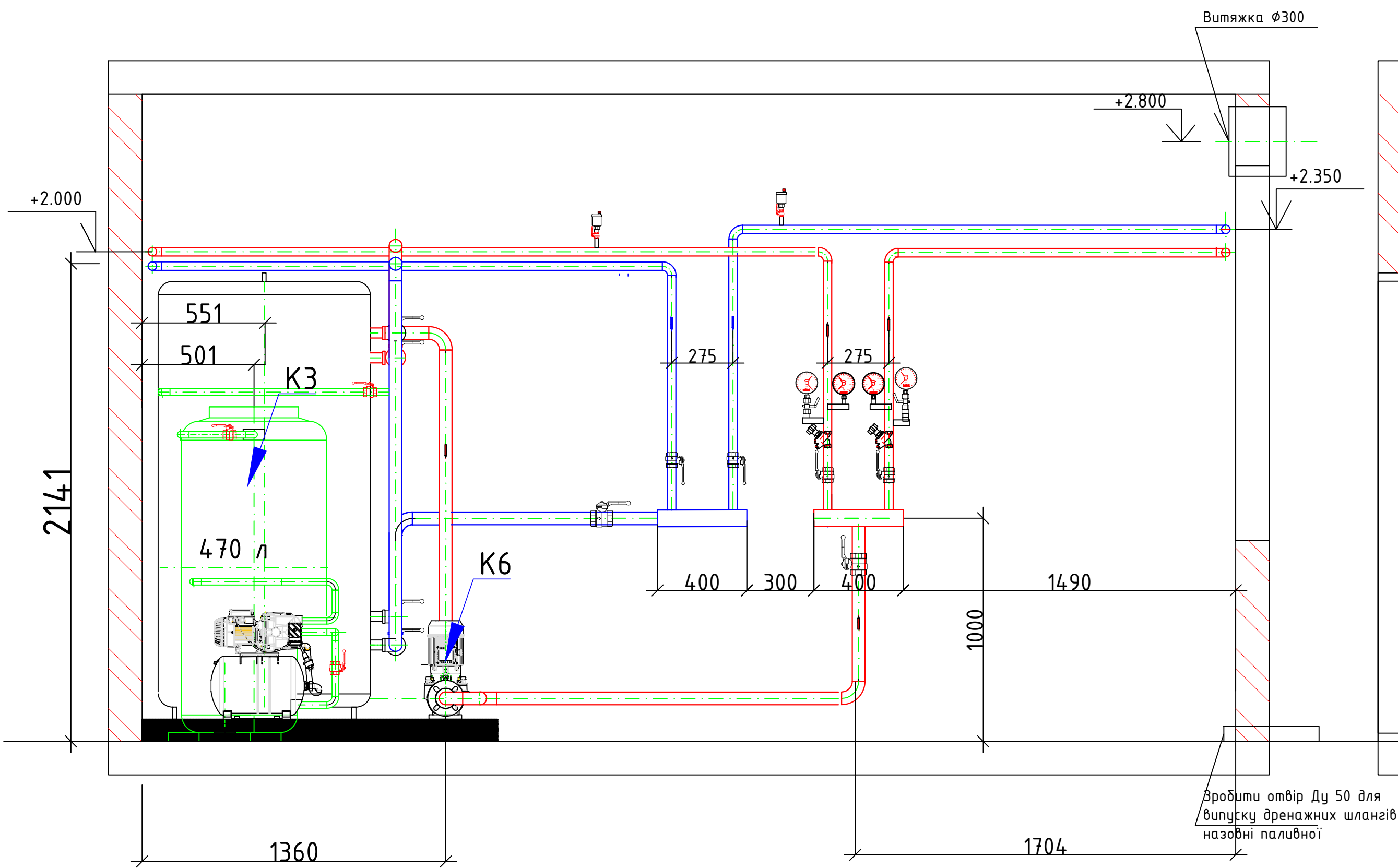
Розріз 1 -1
