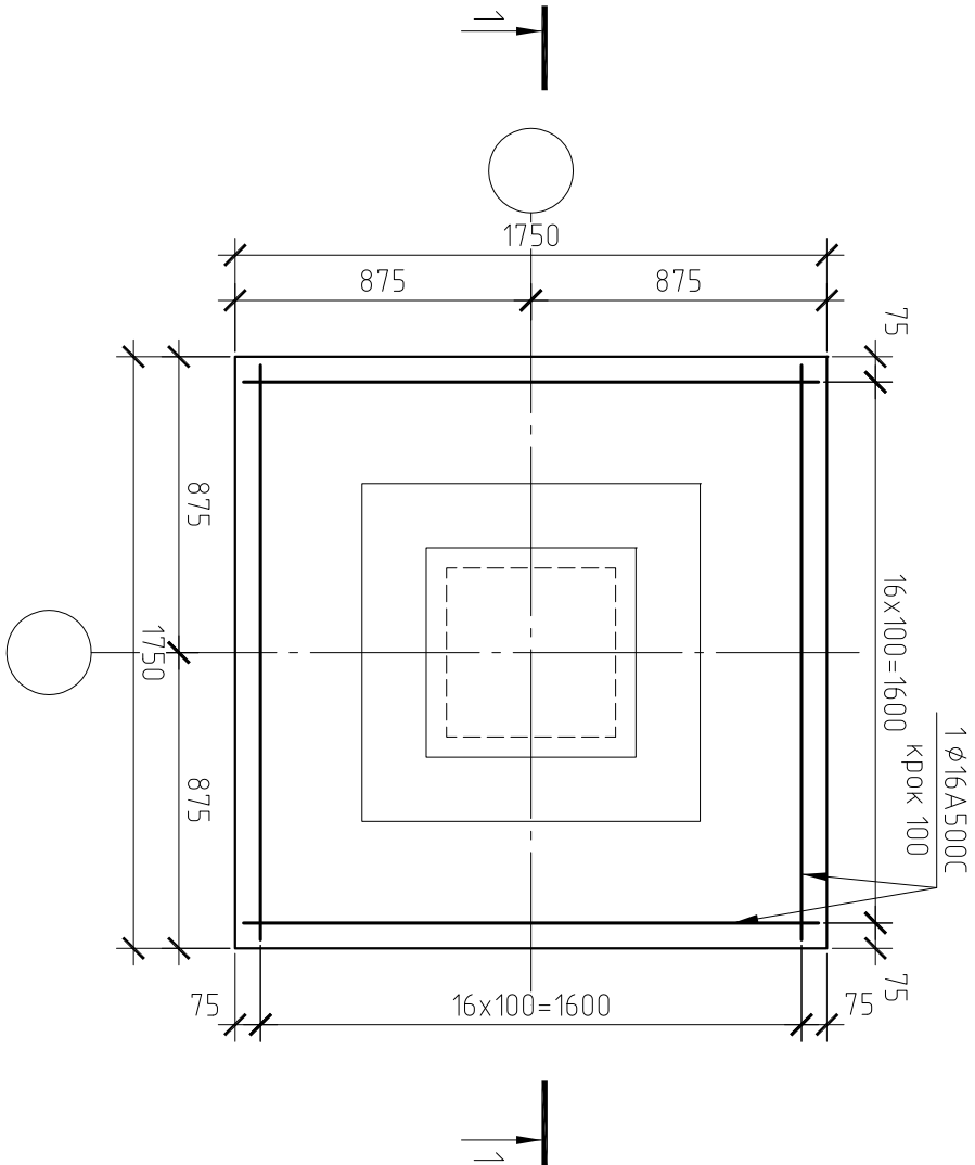
Фундамент ФМ-1
