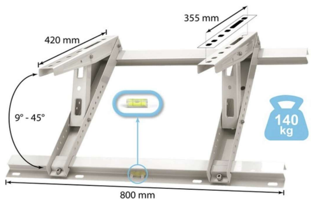
Кронштейн для зовнішнього блоку на дах з нахилом
