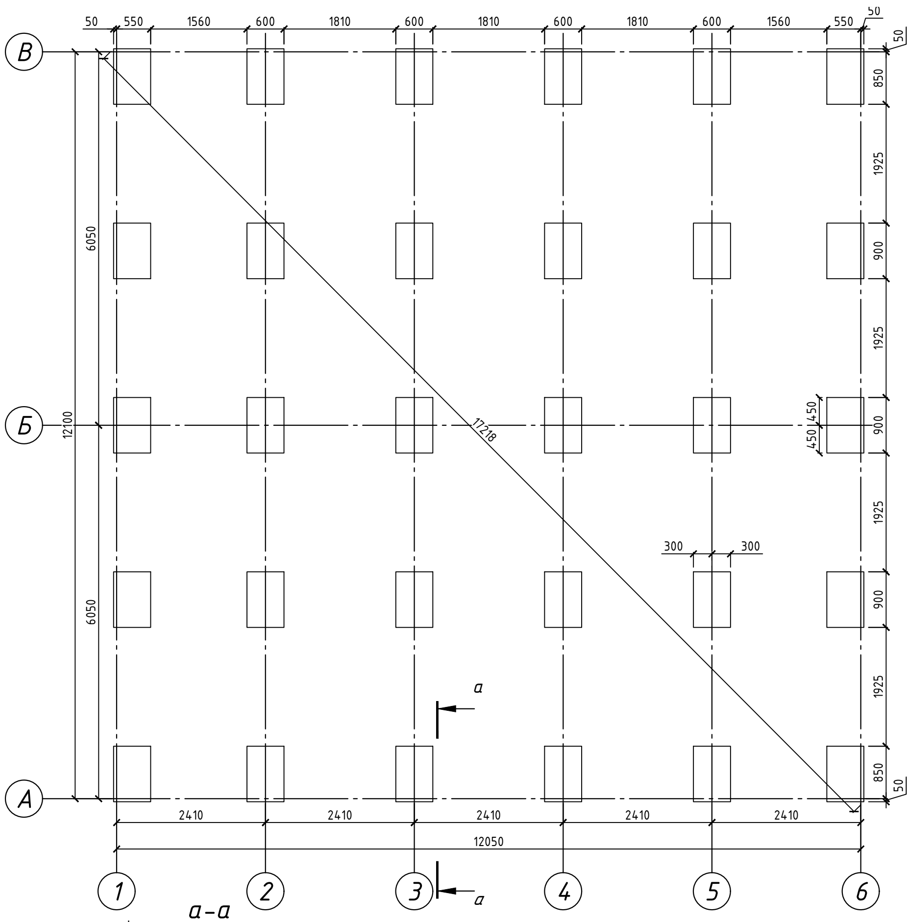
Схема розташування фундаментних блоків
