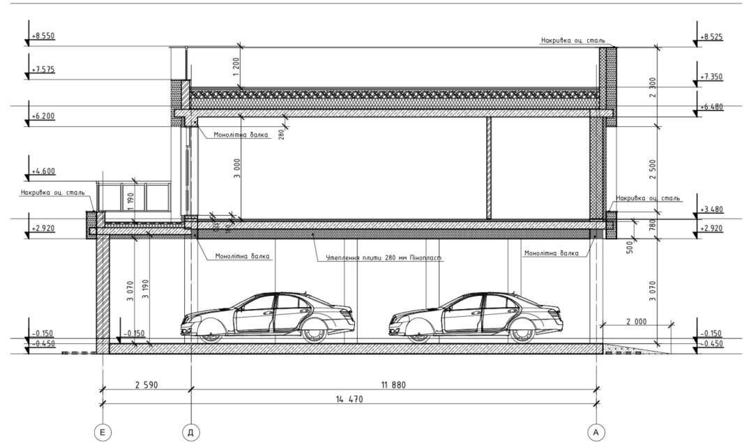
Розріз 4-4
