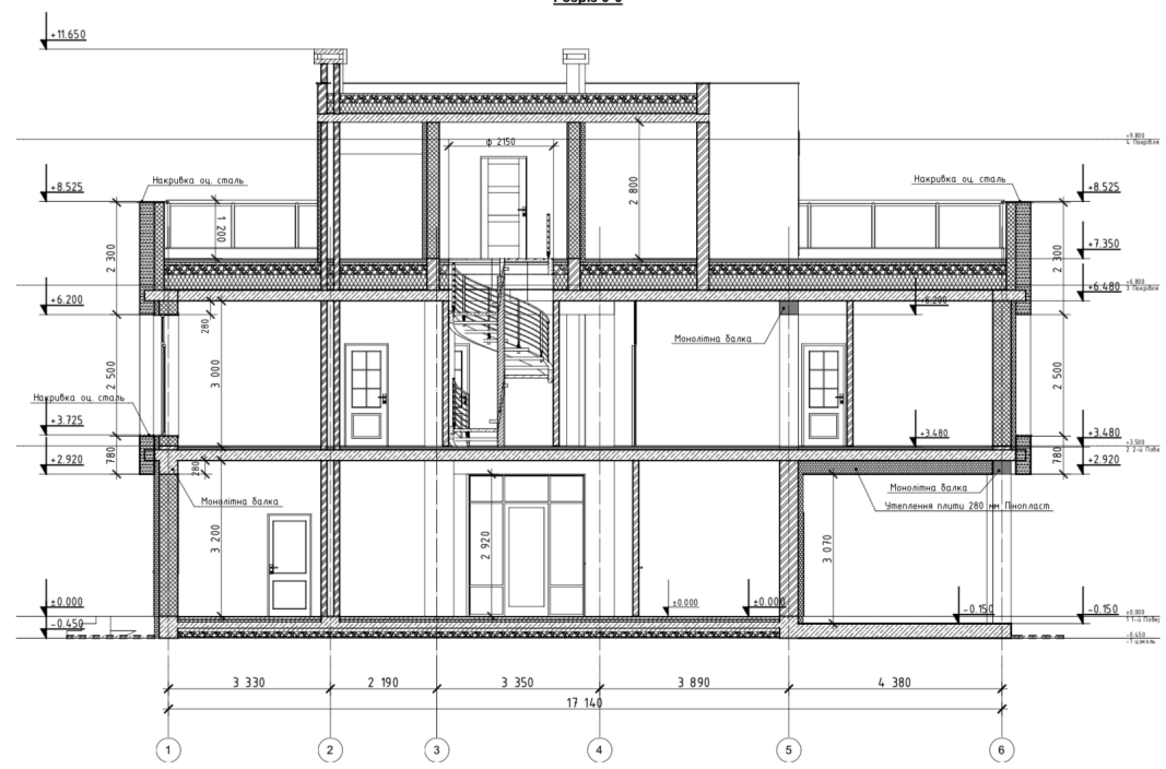
Розріз 6-6
