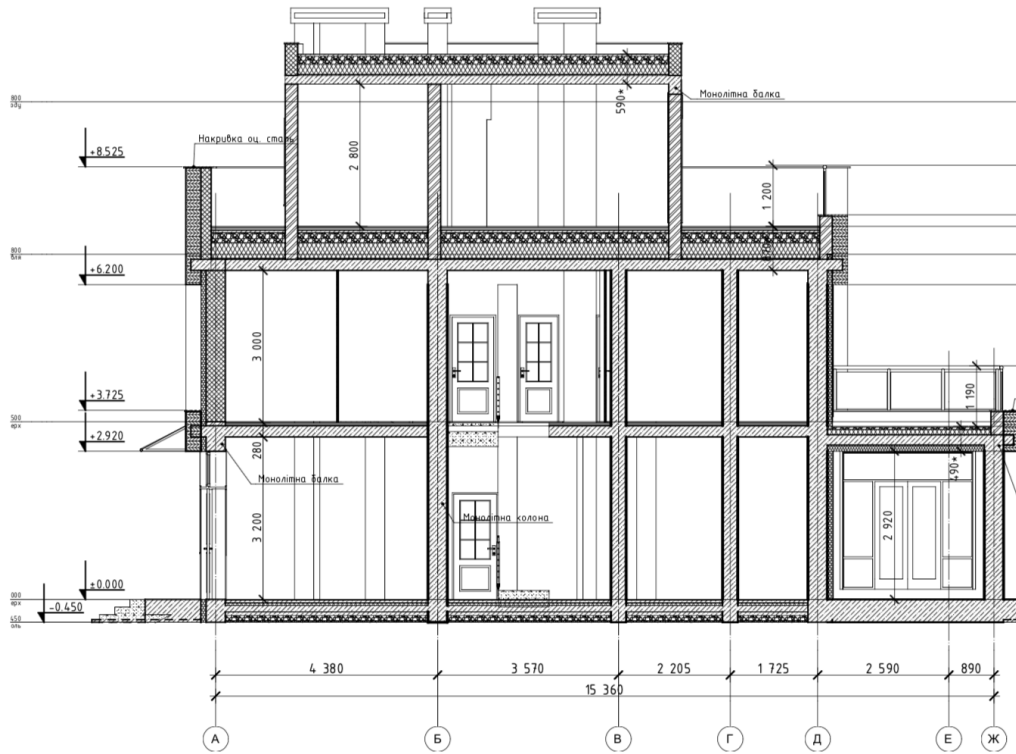
Розріз 5-5
