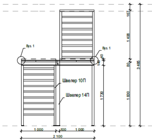
Розріз 1-1
