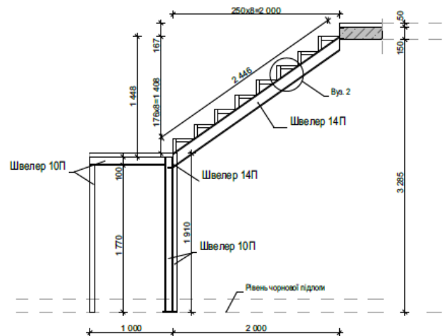
Розріз 2-2
