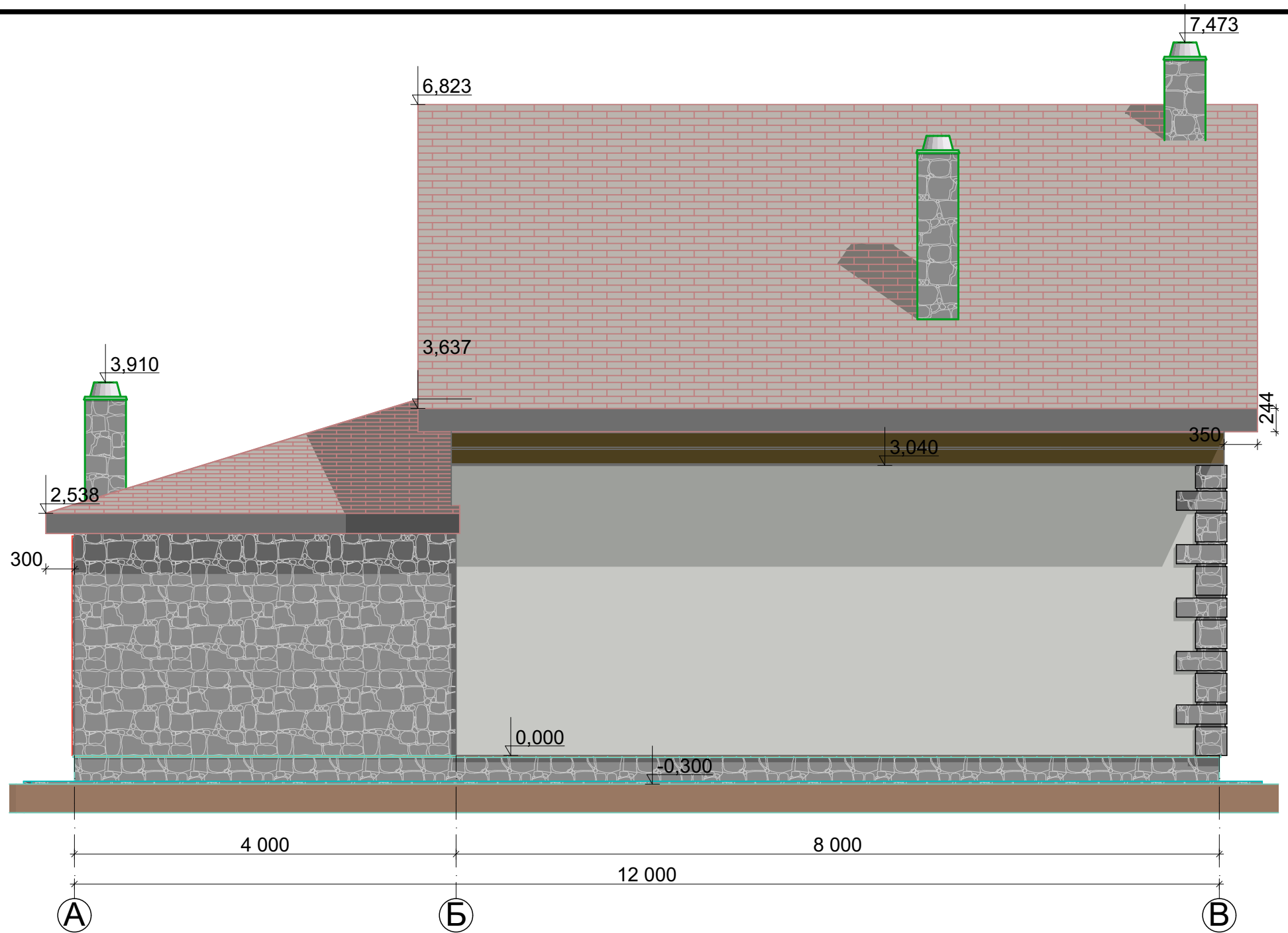
Фасад в осях А-В
