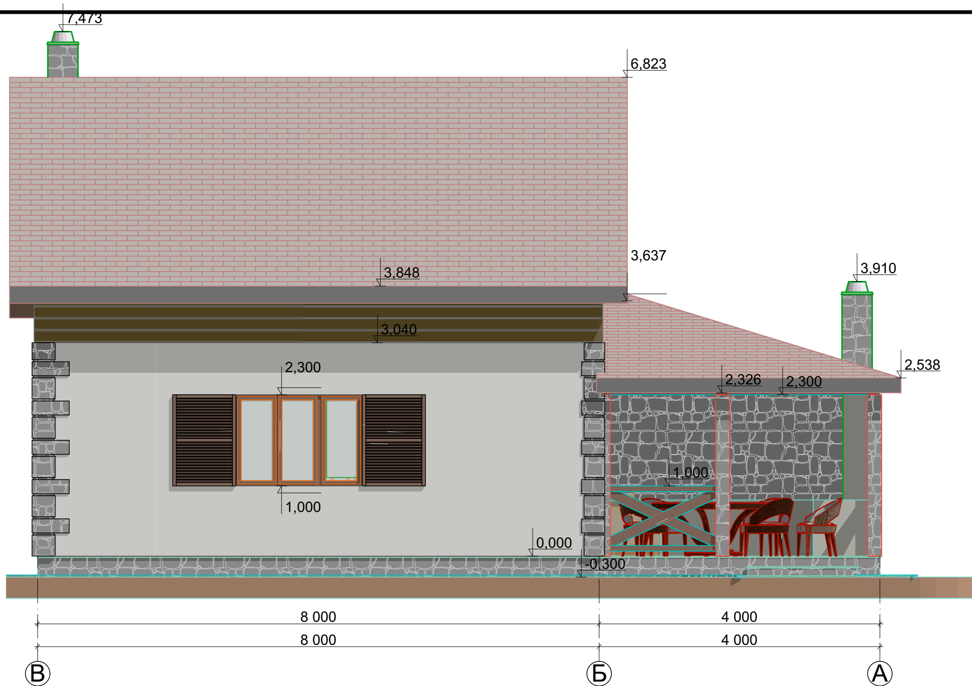
Фасад в осях В-А
