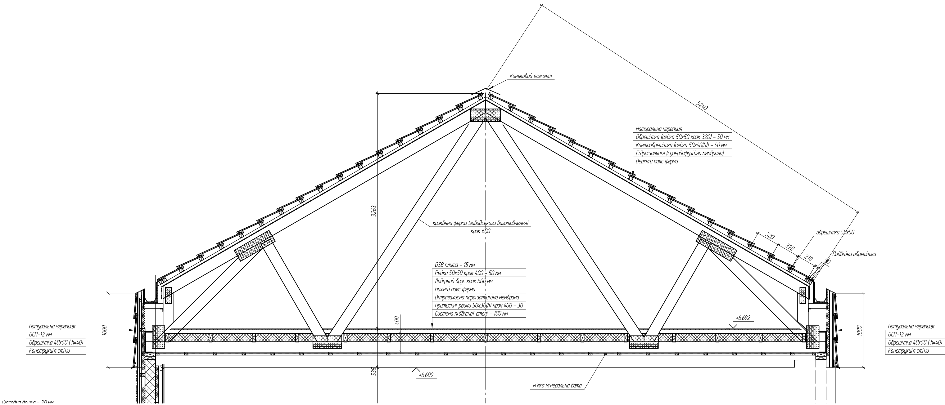
Конструктивний поперечний розріз будинку
