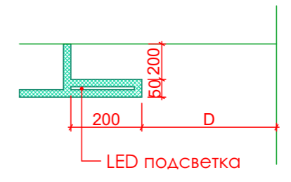
Разрез 3-3
