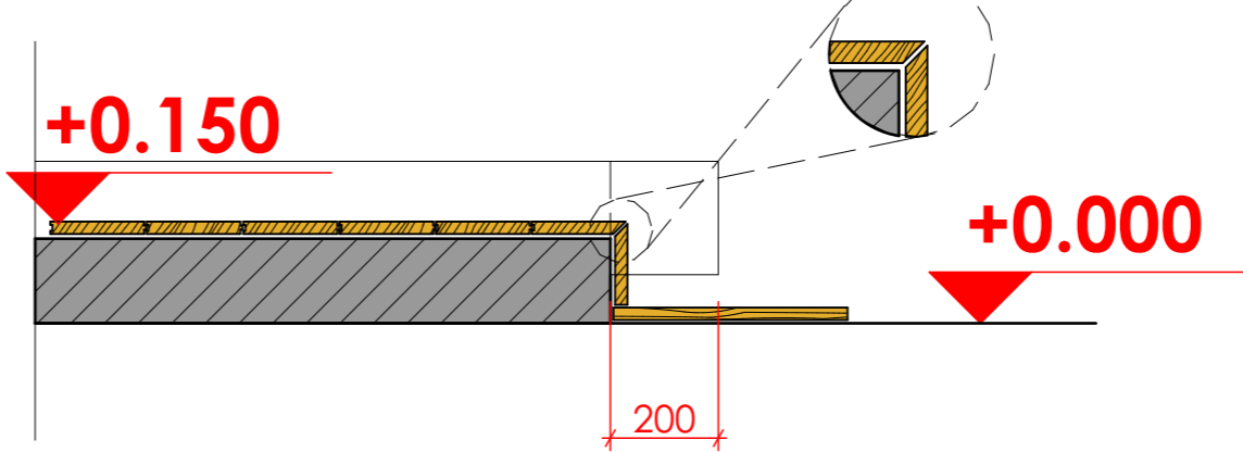
узел 2 прирезка паркета
