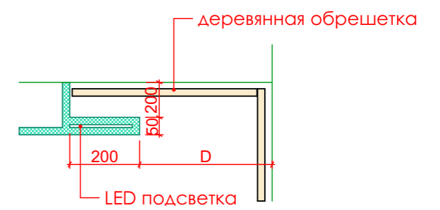
Разрез 4-4
