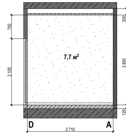
Стіна D-A
