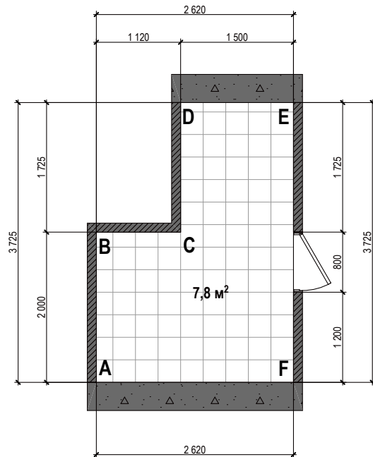
План великої гардеробної
