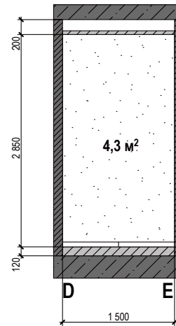
Стіна D-E
