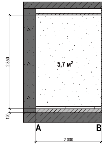
Стіна А-В
