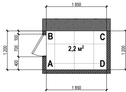
План гостьового санвузла
