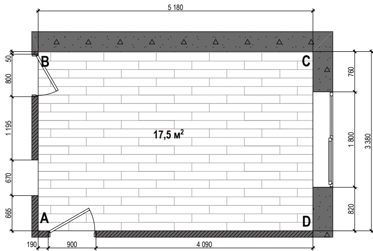
План спальні батьків
