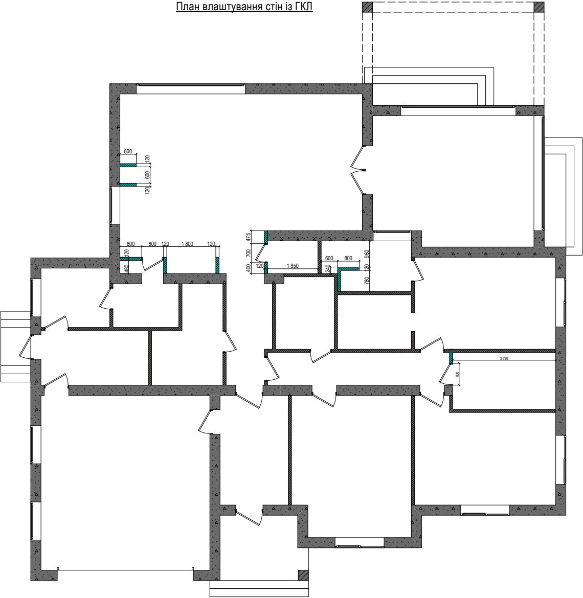
План влаштування стін із ГКЛ
