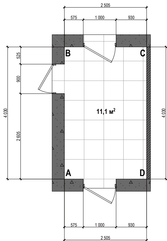
План тамбура
