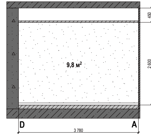
Стіна D-A
