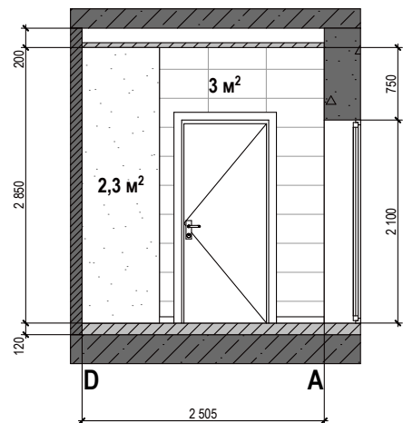
Стіна D-A
