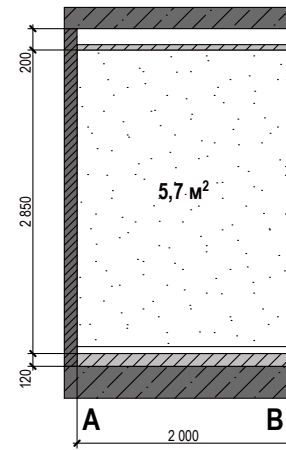
Стіна A-B
