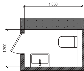
План сантехнічних приладів
