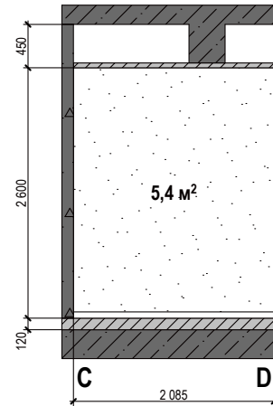
Стіна С-Д
