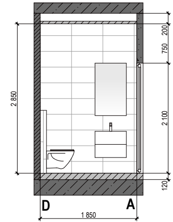
Стіна D-A
