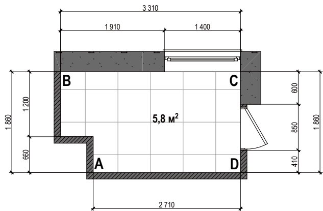
План санвузла батьків
