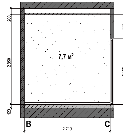
Стіна B-C
