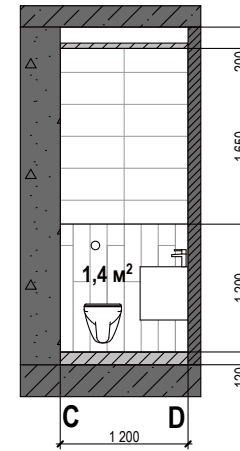
Стіна С-Д
