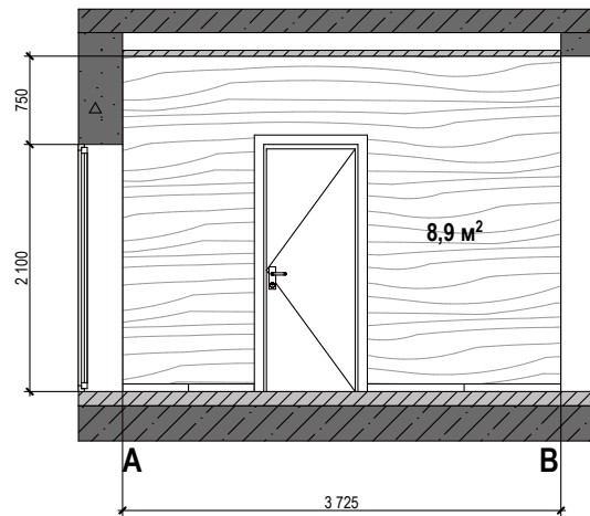
Стіна А-В
