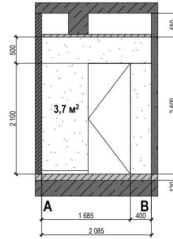
Стіна А-В
