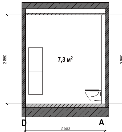
Стіна D-A
