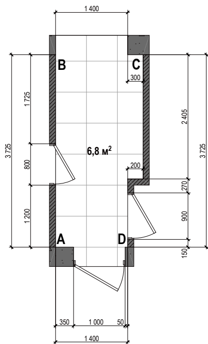
План холу
