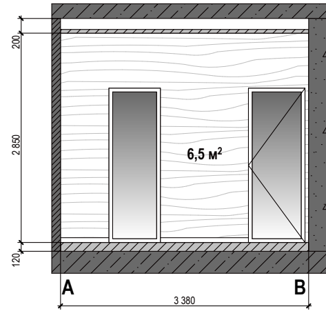
Стіна А-В
