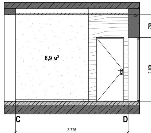
Стіна С-Д
