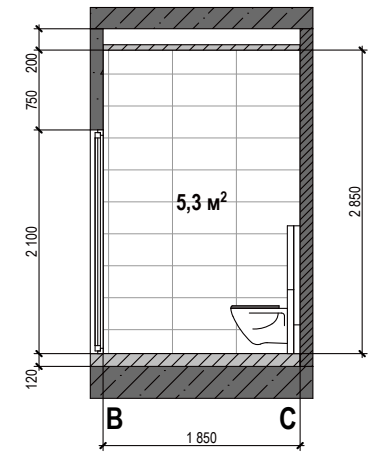
Стіна В-С
