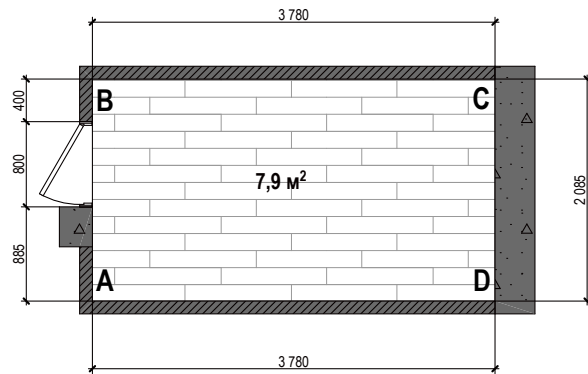
План дитячої гардеробної
