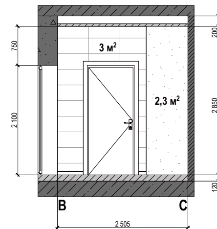
Стіна В-С
