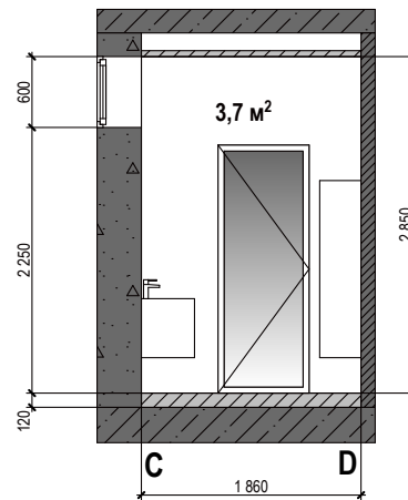
Стіна С-Д
