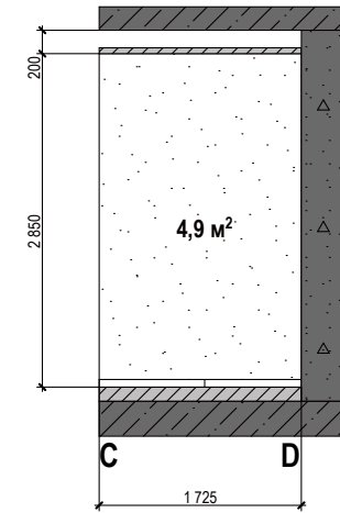
Стіна С-Д
