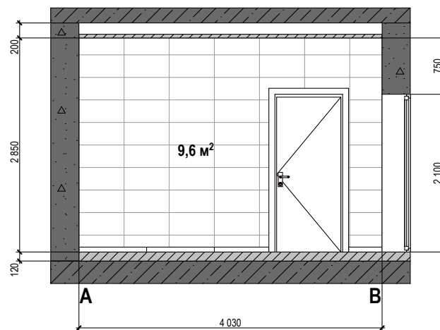
Стіна А-В
