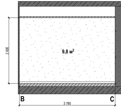
Стіна В-С
