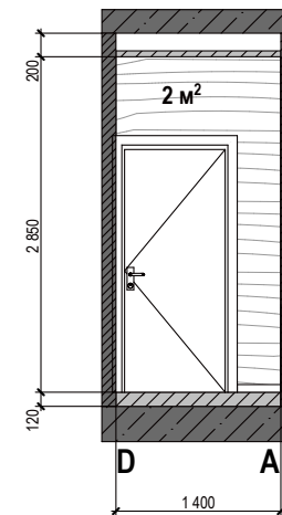
Стіна D-A
