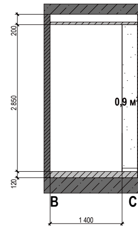
Стіна В-С
