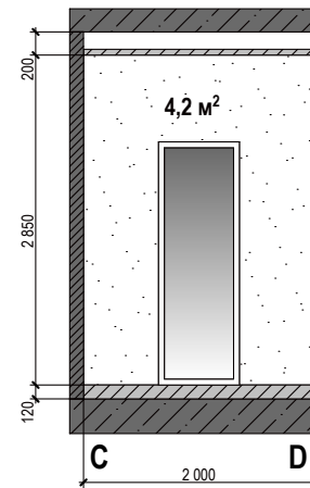
Стіна C-D
