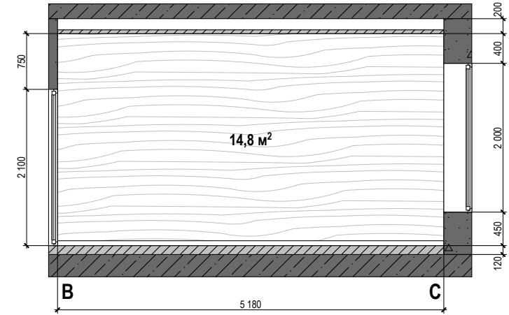
Стіна В-С
