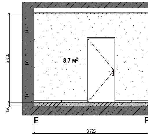
Стіна E-F
