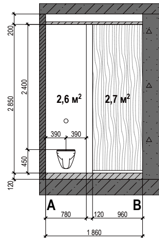
Стіна С-Д
