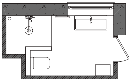
План сантехнічних приладів
