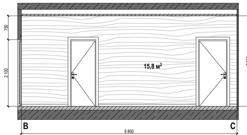
Стіна В-С
