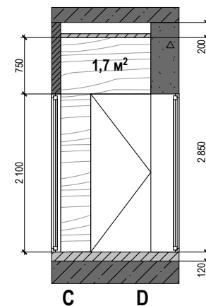
Стіна С-Д
