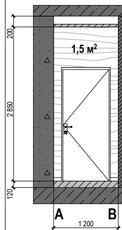
Стіна А-В
