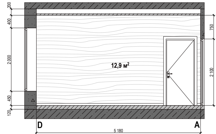
Стіна D-A
