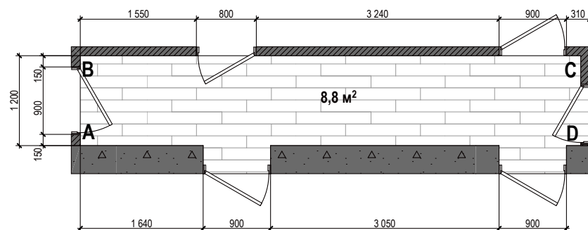
План коридору
