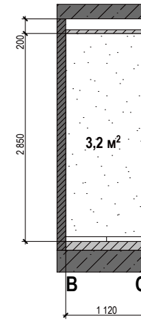
Стіна В-С
