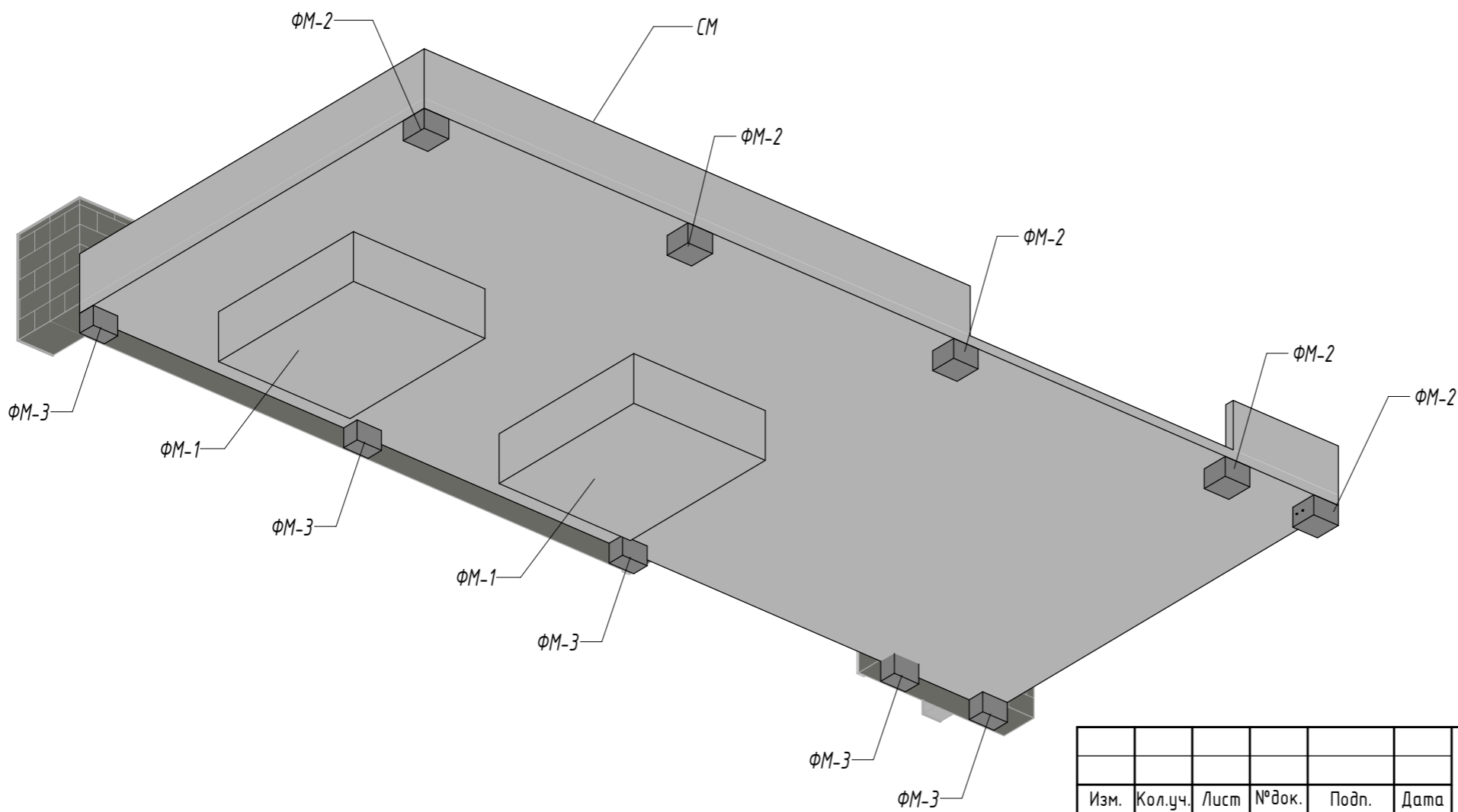
Плита Вид 2 (Вид снизу)
