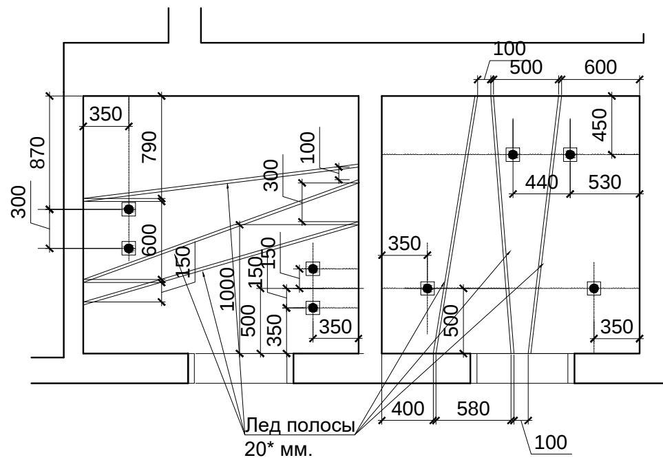
Сан. узлы 1 этажа. План потолка.
