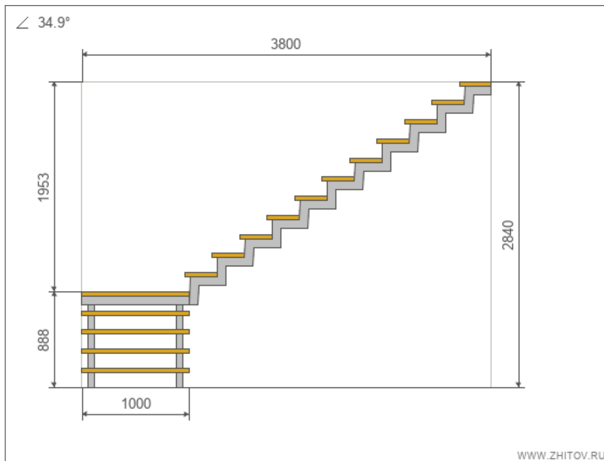
Общий чертеж лестницы
