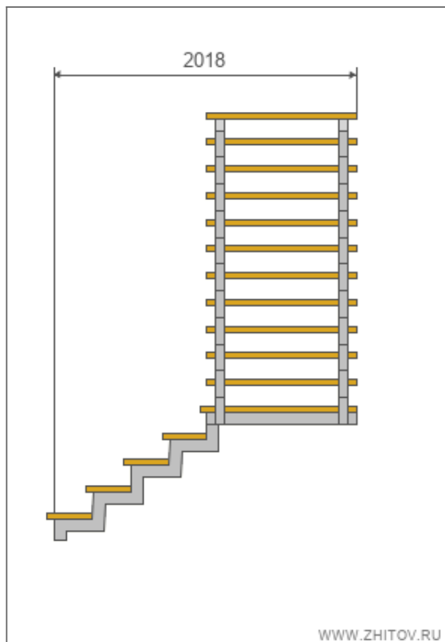
Вид спереди
