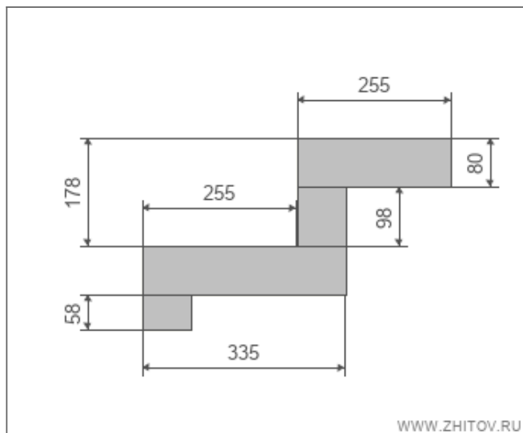
Размеры деталей тетивы
