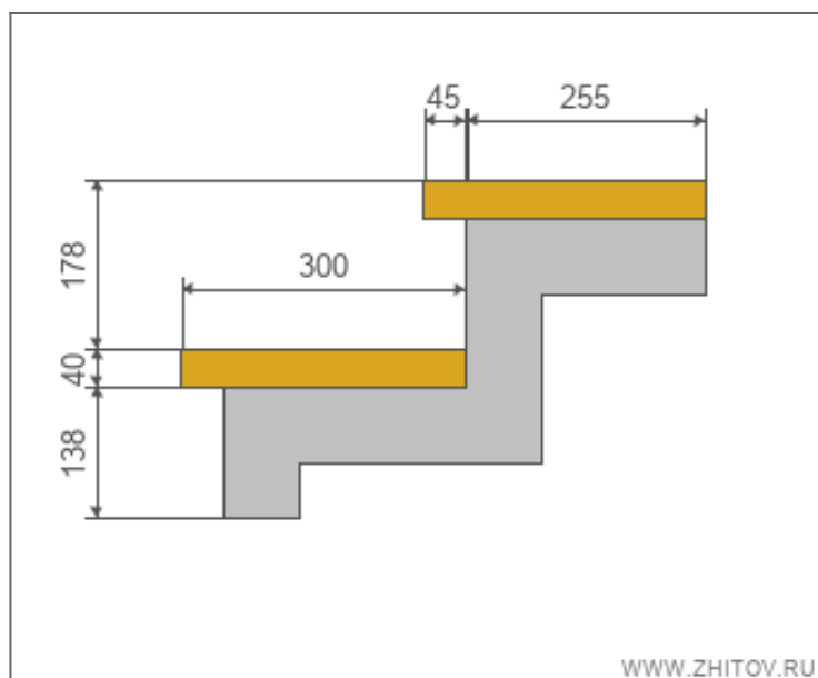
Размеры ступеней
