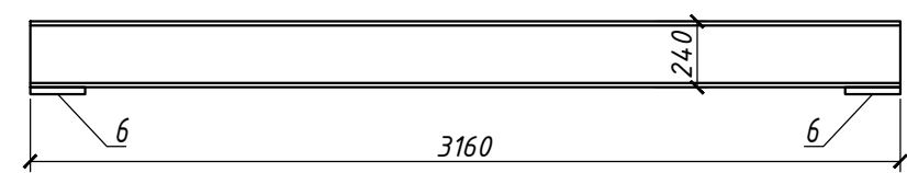
Балка металева Б2
